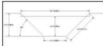
Gambar 4. Dimensi Saluran Terbuka 3
