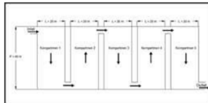
Gambar 7. Dimensi Kolam Pengendapan
