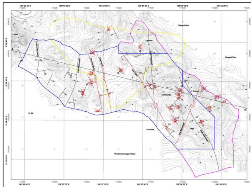
Gambar 5. Peta struktur geologi di area extension
