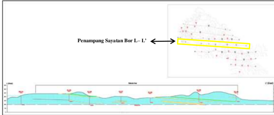
Gambar 17. Penampang bor sayatan L - L'
