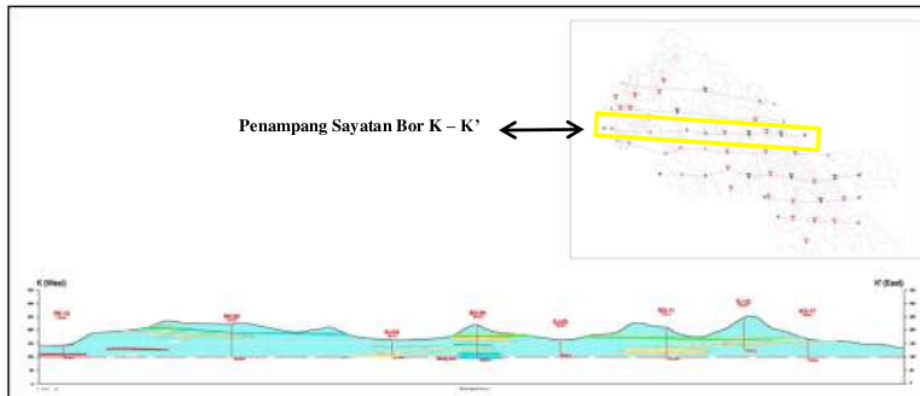
Gambar 16. Penampang bor sayatan K - K'
