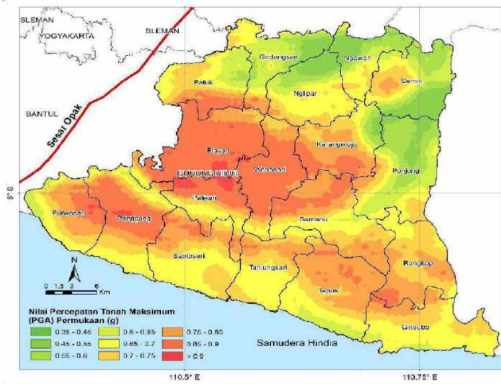
ambar 12. Peta PGA permukaan di Kabupaten Gunungkidul
