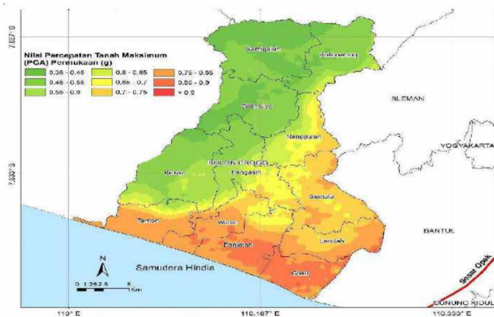
Gambar 10. Peta PGA Permukaan di Kabupaten Kulonprogo
