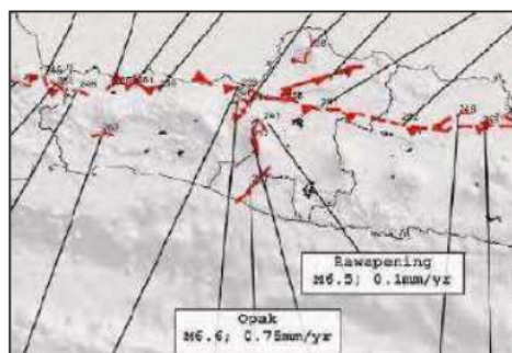
Gambar 2. Sesar Lokal di DIY dan Sekitarnya (PUSGEN 2017)
