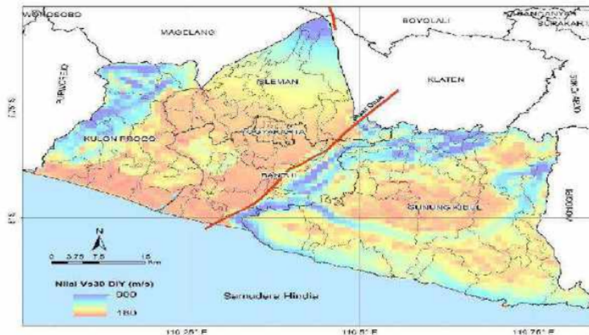
Gambar 6. Peta Vs30 di Daerah Istimewa Yogyakarta
