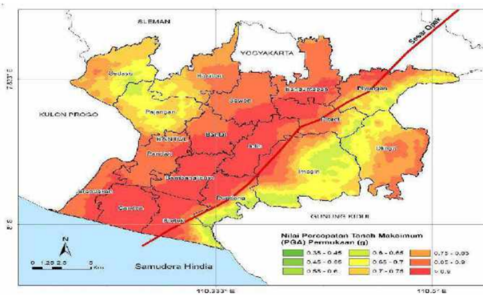
Gambar 8. Peta PGA permukaan di Kabupaten Bantul
