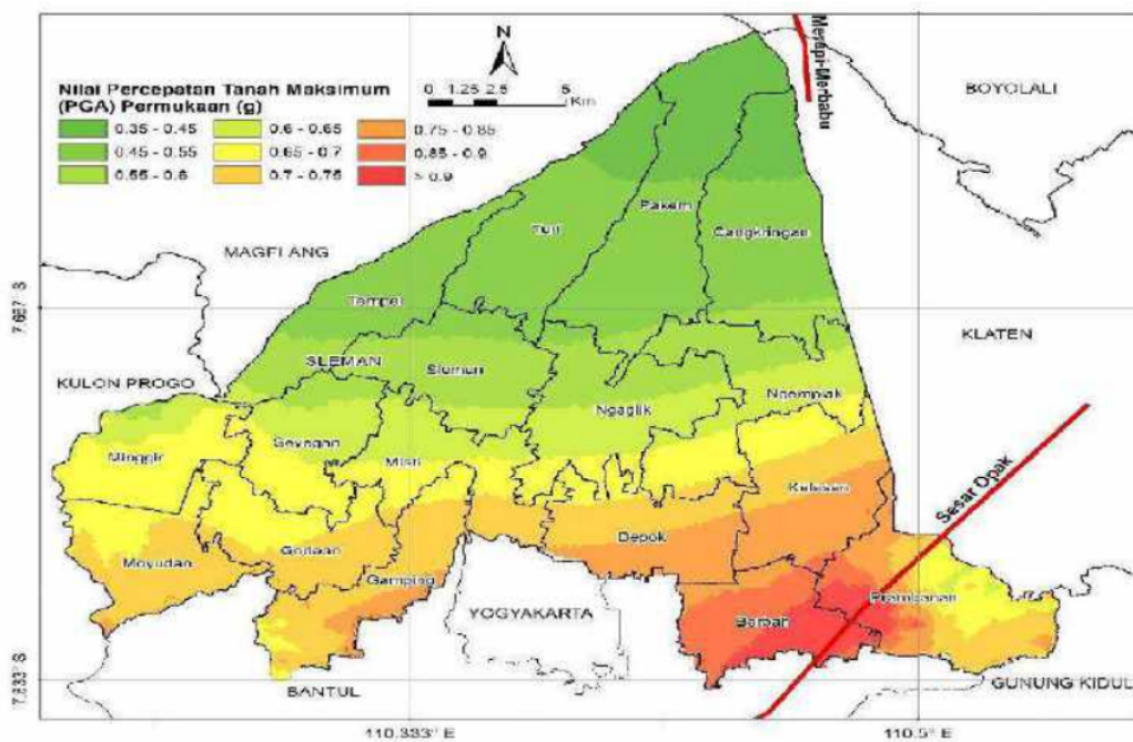
Gambar 11. Peta PGA permukaan di Kabupaten Sleman
