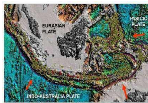
Gambar 1. Kondisi Tektonik Indonesia (Badan Geologi, ESDM)
