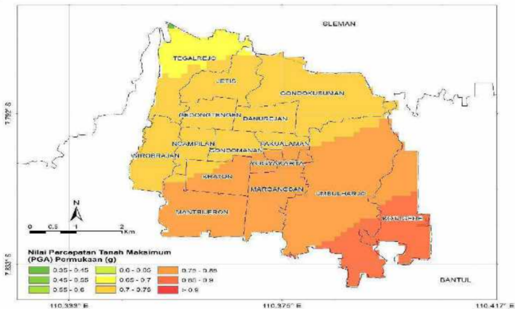
Gambar 9. Peta PGA permukaan di Kota Yogyakarta
