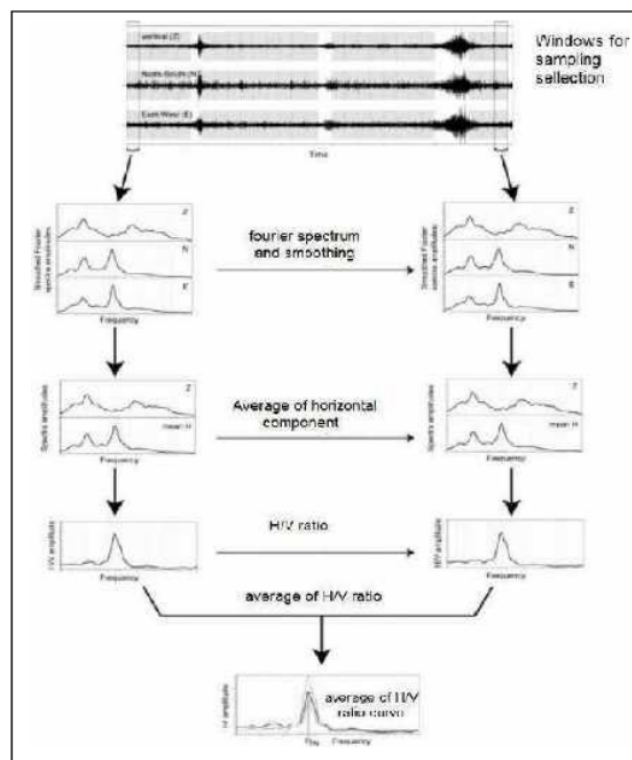
Gambar 4. Prosedur pengolahan data metode HVSR (sesame 2004)
