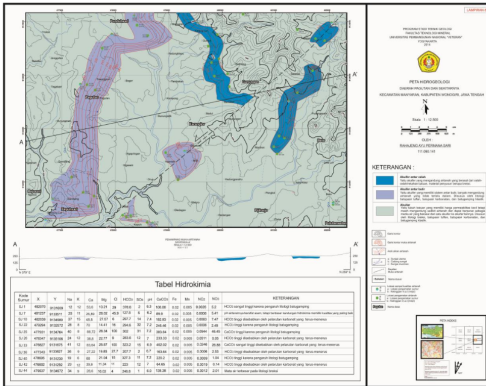
Gambar 3. Peta hidrogeologi daerah penelitian (tanpa skala)
