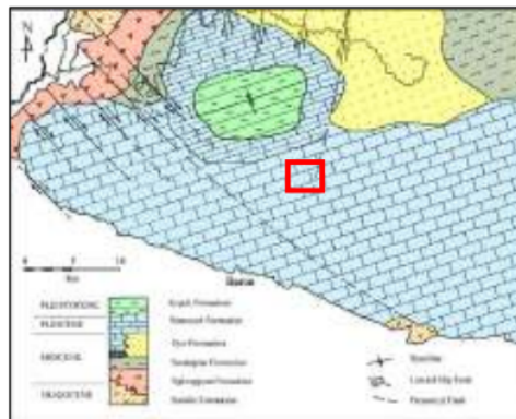
Figure 2 Geological Map of Gunung Sewu, Gunung Kidul (Kusumayudha et al., 2015)
