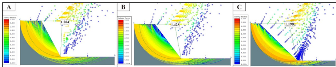
Gambar 19 (A) Hasil analisis kestabilan lereng 1 (B) Hasil analisis kestabilan lereng 2 (C) Hasil analisis kestabilan lereng 3
