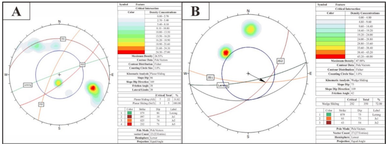
Gambar 24. Hasil Analisis Kinematik lereng
