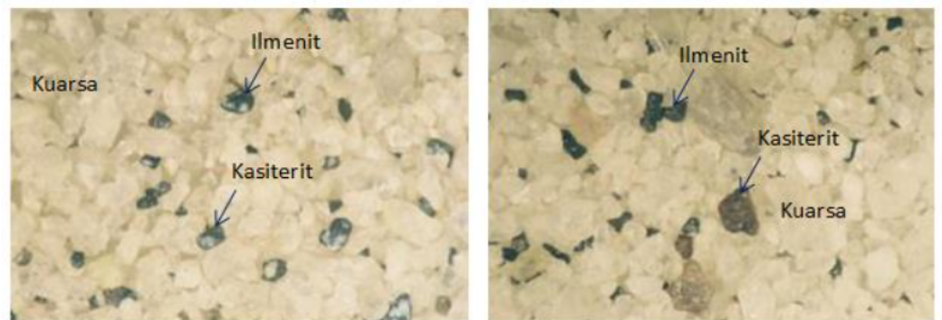
Gambar 4.5. Mineral yang hadir kasiterit, ilmenit, zircon, turmalin, muskovit dan mineral kuarsa pada LP12 (kiri) dan LP13 (kanan).
