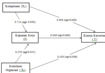
Gambar 2. Model Analisis Jalur
