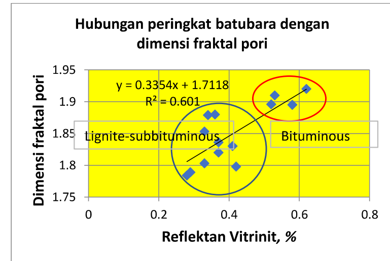
Gambar 21. Hubungan antara dimensi fractal dengan peringkat batubara
