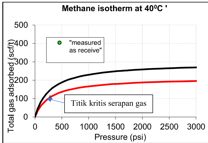
Gambar 15. Kurva antara tekanan dan volume serapan gas
