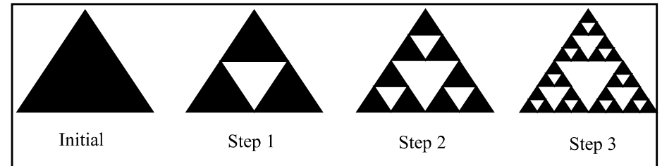
Gambar 2. Model Segitiga Sierpinski (Kusumayudha, 2005)
