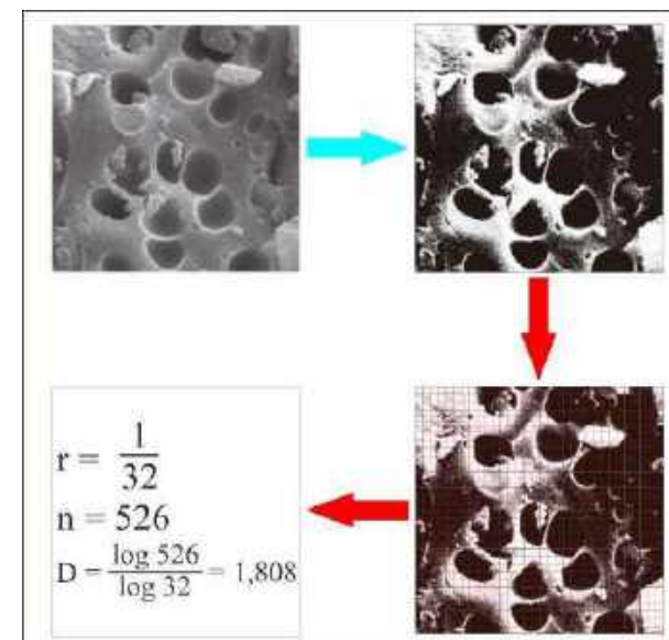
Gambar 7. Perhitungan manual metode box counting dengan r = \frac{1}{32}
