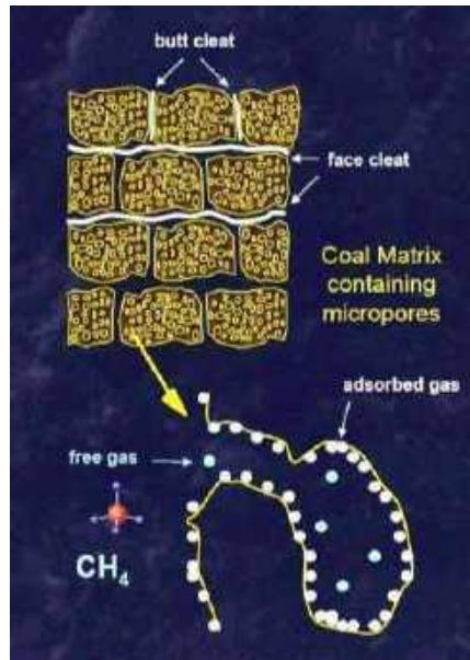
Gambar 13. Keberadaan gas pada pori-pori matrik batubara
