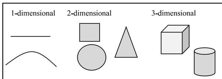
Gambar 3. Bentuk Geometri Euclidean
