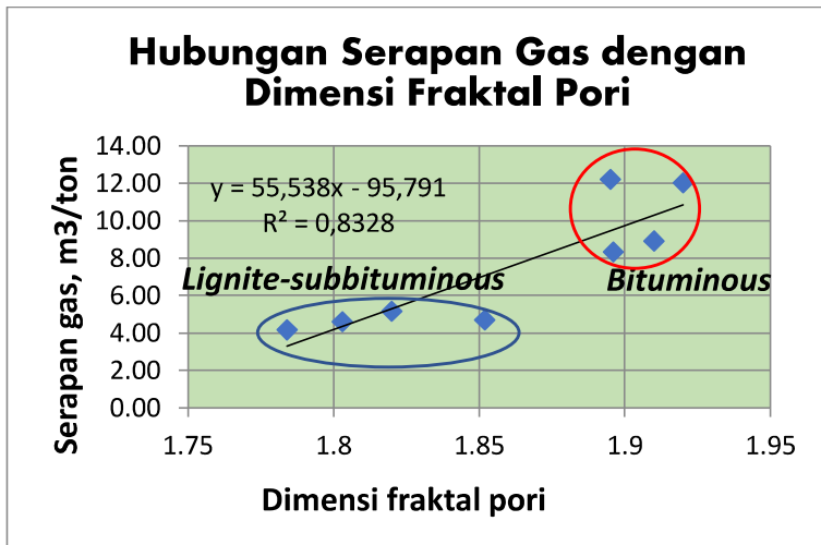
Gambar 22. Hubungan antara serapan gas metana dengan dimensi fractal.
