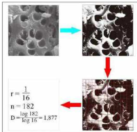
Gambar 6. Perhitungan manual metode box counting dengan
