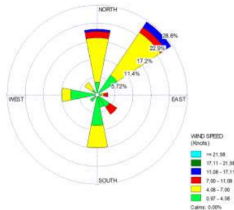
Gambar 2. Windrose daerah penelitian tahun 2010 – 2019
