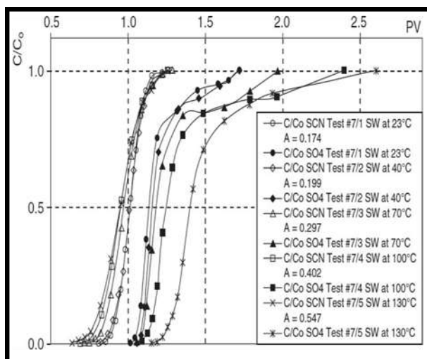
Gambar 1.2. Retensi Ion \text{SO}_4^{2-} dan \text{SCN}^- Pada Temperatur Berbeda (Strand et al., 2006) (Sheng, James. 2010)
