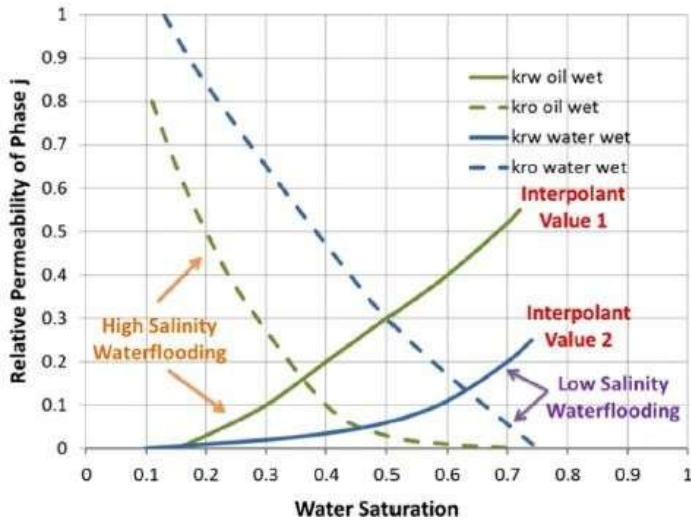
Gambar 3.2 Kurva Permeabilitas Relative
