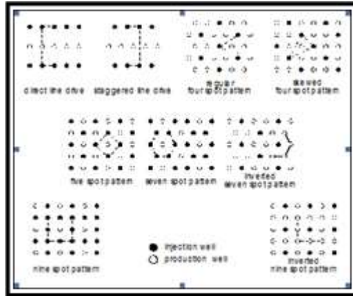
Gambar 1.4. Pola-Pola Sumur Injeksi-Produksi (Gomaa, E.E..1995)
