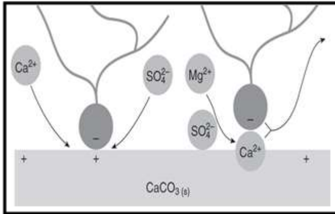
Gambar 1.1. Mekanisme MIE Saat Ion Mg^{2+} dan SO_4^{2-} Aktif Pada Temperatur Tinggi (Sheng, James. 2010)
