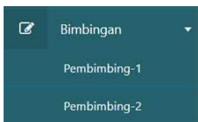
Gambar 3.8 Menu Bimbingan
