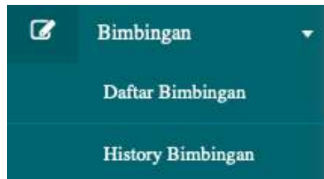
Gambar 5.13 Menu Bimbingan
