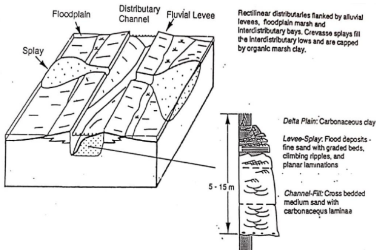
Gambar 5. Model sub-lingkungan pengendapan delta plain [1]
