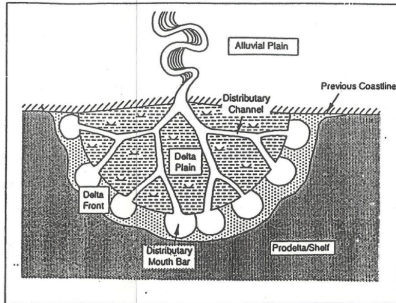
Gambar 5. Komponen dasar lingkungan pengendapan delta [1]
