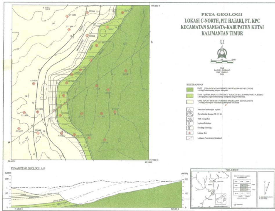
Gambar 3. Peta Geologi Daerah penelitian Sangatta Kalimantan Timur [5]
