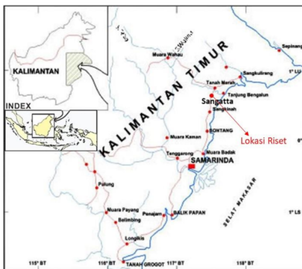
Gambar 1. Lokasi Riset Sangatta, Kalimantan Timur
