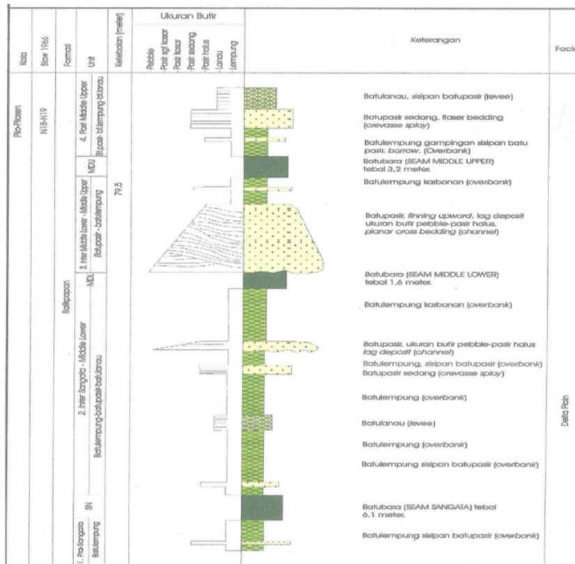
Gambar 2. Stratigrafi Rinci Daerah penelitian Sangatta Kalimantan Timur [5]
