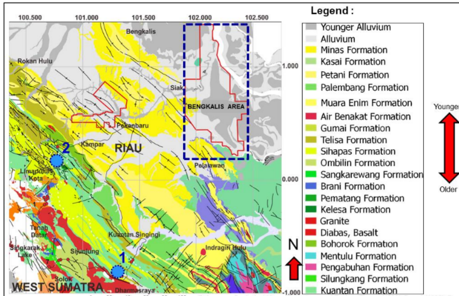
Gambar 5. Lokasi observasi dan Kavling target penelitian. (Peta Geologi Lembar Pekanbaru dan Tanjung Pinang (1980), Dumai (1982), Rengat (1994) and Solok (1995) From PPPG (Pusat Penelitian dan Pengembangan Geologi)).
