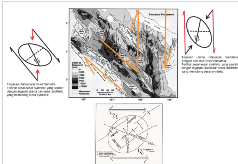
Gambar 6. Penggunaan Konsep Harding (1973) dalam penentuan stress utama lokasi telitian.
