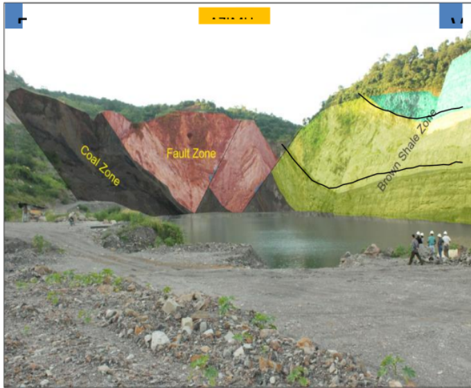
Gambar 4. Lokasi Pengamatan 1 dengan sesar turun yang mempunyai strike relatif ke tenggara dan dip relatif ke barat daya.
