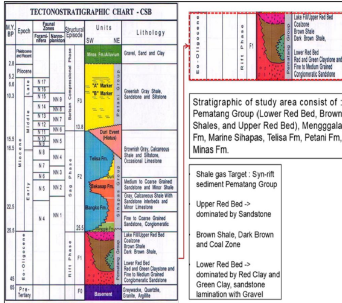
Gambar 3. Tektonostratografi Cekungan Sumatra Tengah (Heidrick dan Aulia, 1993; Kelompok Pematang ditunjukkan pada lingkaran merah, dalam Sunardi, 2015).
