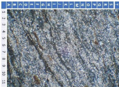
Gambar 6. Kenampakan mikroskospis shale
