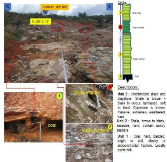
Gambar 5. Pembagian fasies shale unit-1, 2 dan 3.
