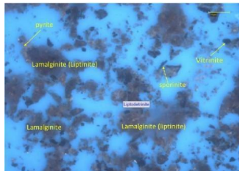
Gambar 9. Kenampakan mikroskopis organik shale di Desa Batubalang (posisi sinar ultra violet)
