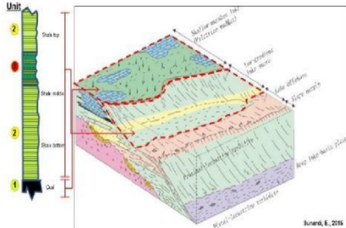
Gambar 7. Fasies pengendapan shale di Desa Batubalang
