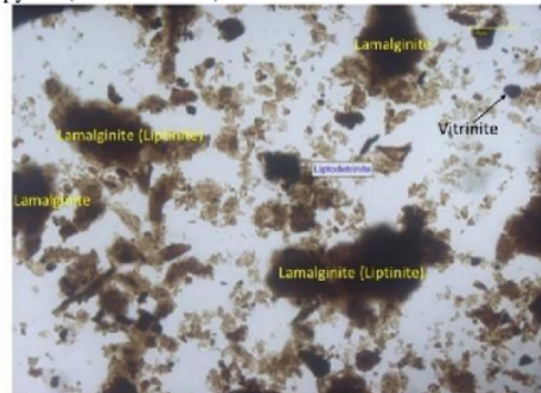
Gambar 8. Kenampakan mikroskopis organik shale di Desa Batubalang (posisi sinar putih)
