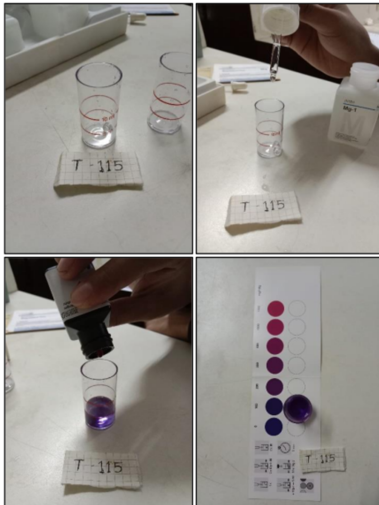
Gambar IV.7. Pengujian Kadar Magnesium Air Formasi
