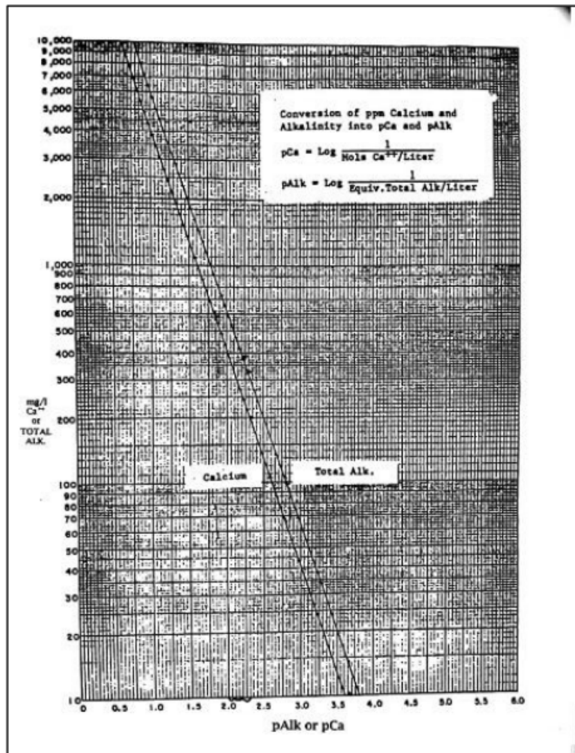
Gambar IV.9. Grafik Nilai pCa dan pAlk pada Berbagai Ion Ca 2+
