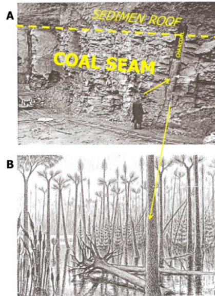
Gambar 10. Rekonstruksi pembentukan charcoal (arang kayu) [7]
