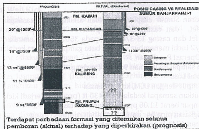
Gambar 1. Ilustrasi Rencana dan Operasi pemasangan Casing Sumur X
