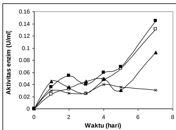
Gambar 4. Aktivitas Enzim pada berbagai Konsentrasi Substrat (g/100ml): (□),6; (■),9; (▲),12; (×), 15.
