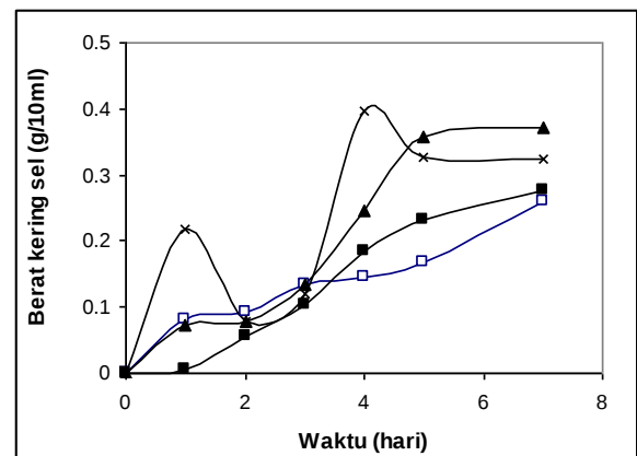
Gambar 3. Berat Kering Sel pada berbagai Konsentrasi Substrat (g/100ml): (□),6; (■),9; (▲),12; (×),15.
