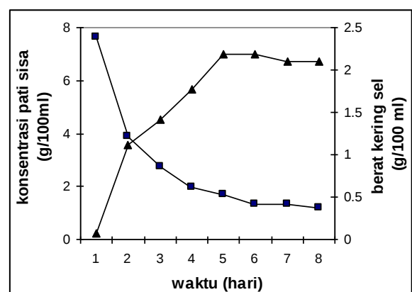
Gambar 7. Berat Kering Sel dan Konsentrasi pati sisa pada Konsentrasi Substrat 9 % dengan pH 6
