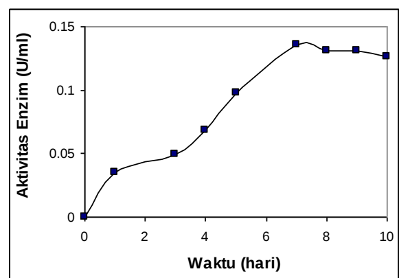
Gambar 8. Aktivitas Enzim pada Konsentrasi Substrat 9 % dengan pH 6
