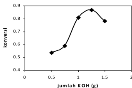
Gambar 4. Hubungan penambahan katalis KOH terhadap konversi
