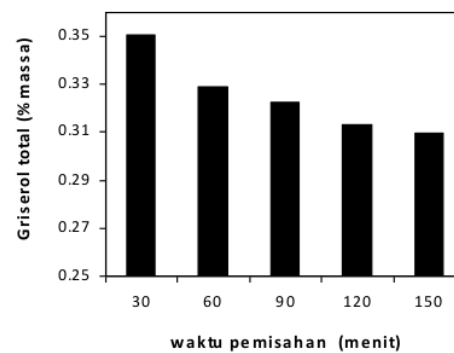
Gambar 5. Hubungan Waktu Pemisahan terhadap Kadar Gliserol Total
