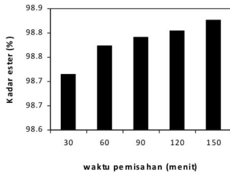
Gambar 6. Hubungan Waktu Pemisahan terhadap Kadar Ester
