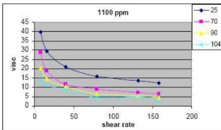
Gambar 5. Viskositas polimer HYBOMAX 4785 konsentrasi 1100 ppm
