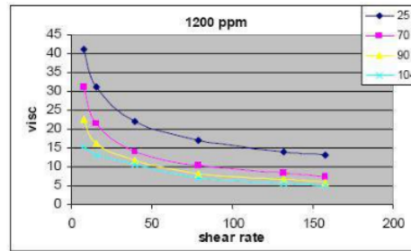
Gambar 6. Viskositas polimer HYBOMAX 4785 konsentrasi 1200 ppm
