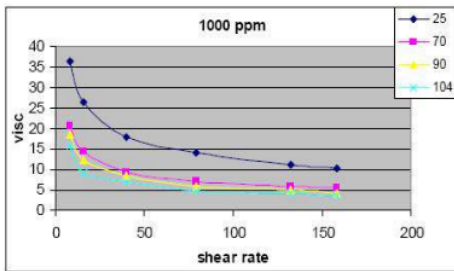
Gambar 4. Viskositas polimer HYBOMAX 4785 konsentrasi 1000 ppm
