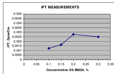
Gambar 3. Grafik hasil pengukuran interfacial tension
