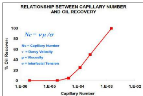
Gambar 1. Pengaruh capillary number terhadap perolehan minyak (After Berger, D., et. al., 2002)
