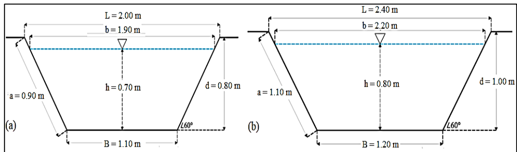
Gambar 3. Desain Saluran Terbuka (a) Dimensi I; (b) Dimensi II
