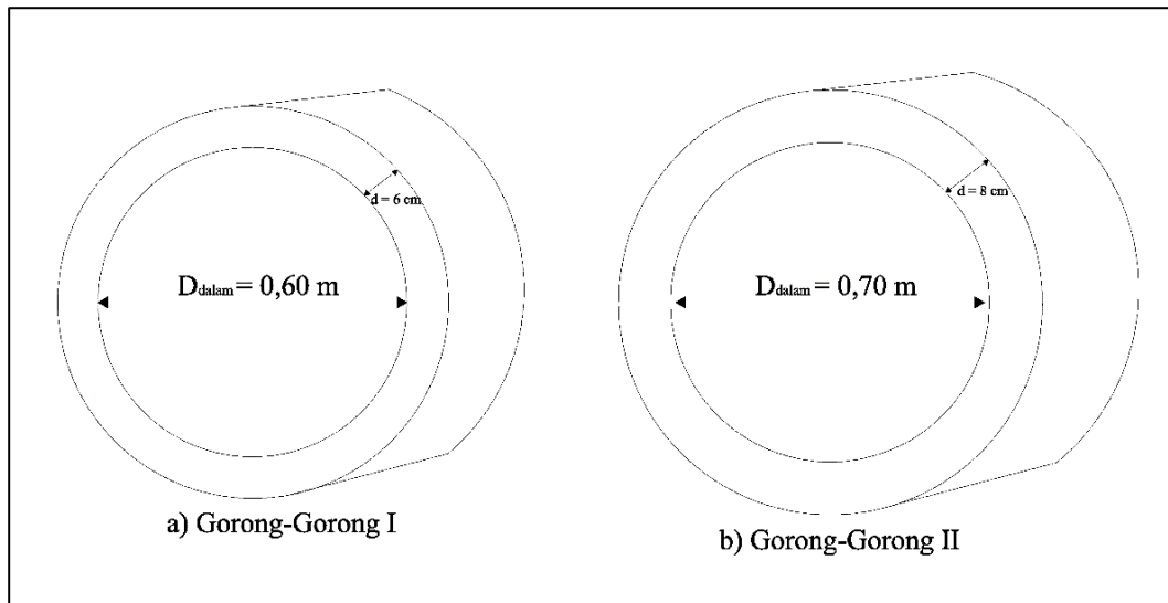
Gambar 4. Dimensi Rancangan (a) Gorong-Gorong I; (b) Gorong-Gorong II
