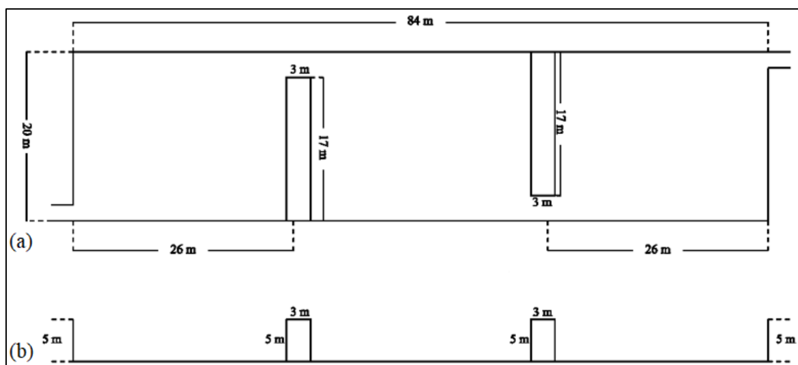
Gambar 5. Dimensi Kolam Pengendapan (a) Tampak Atas (b) Tampak Samping
