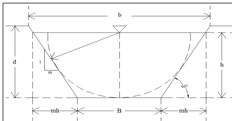
Gambar 2. Bentuk Trapesium dari Open Channel
