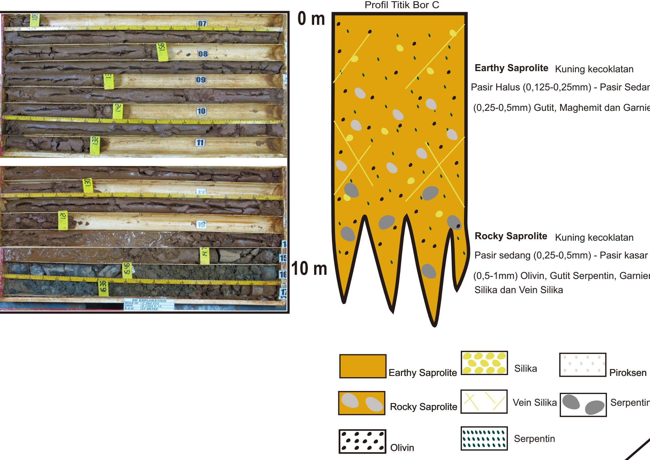
Profil Titik Bor C
