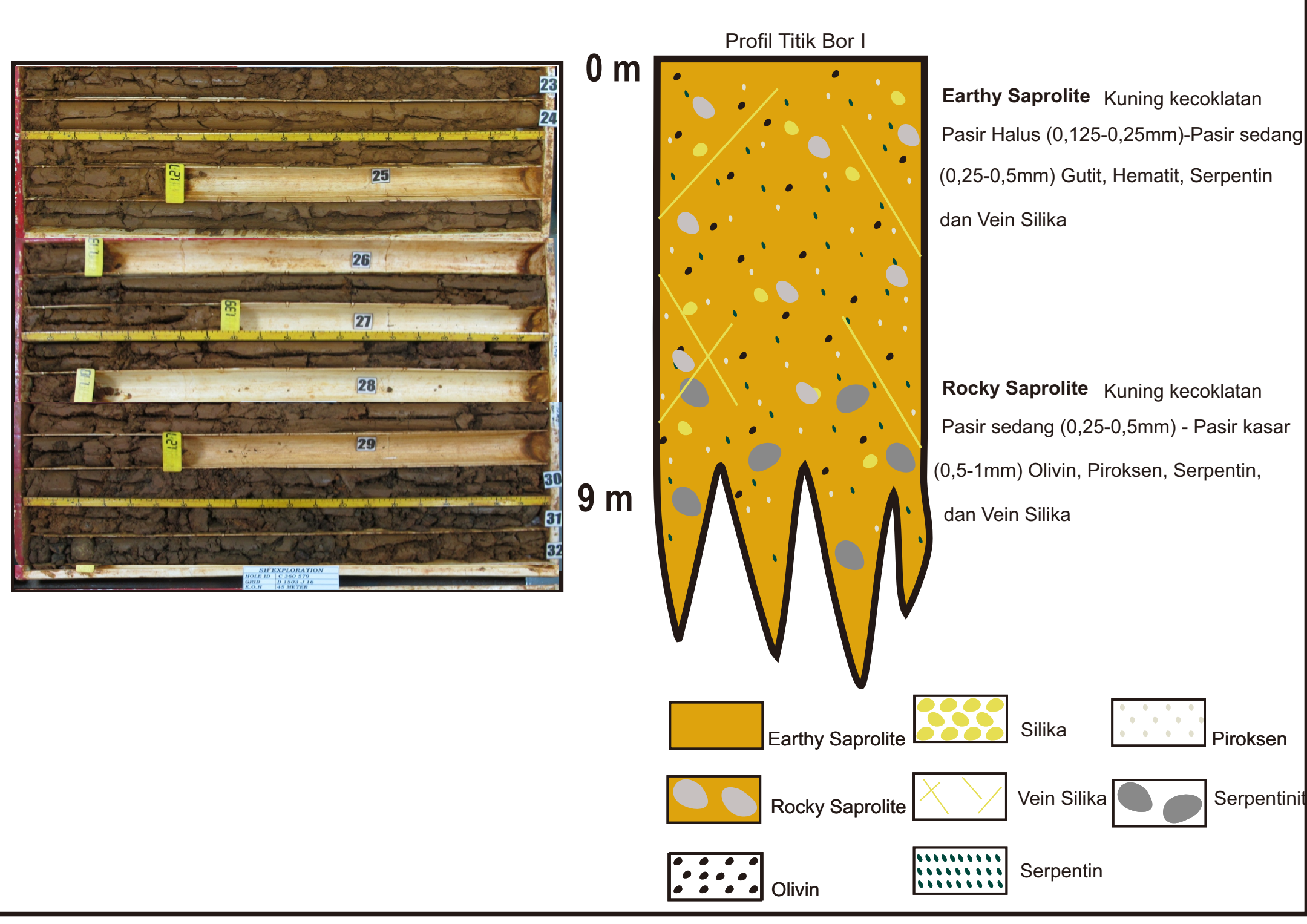
Profil Titik Bor I
