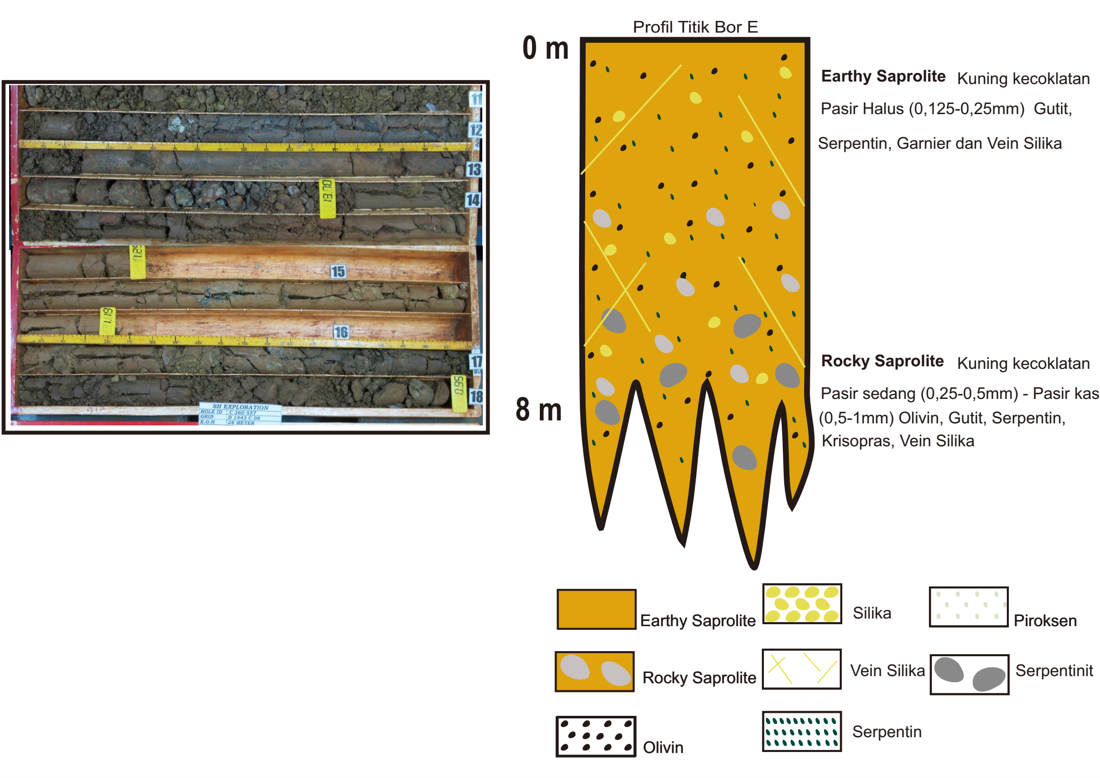
Profil Titik Bor E
