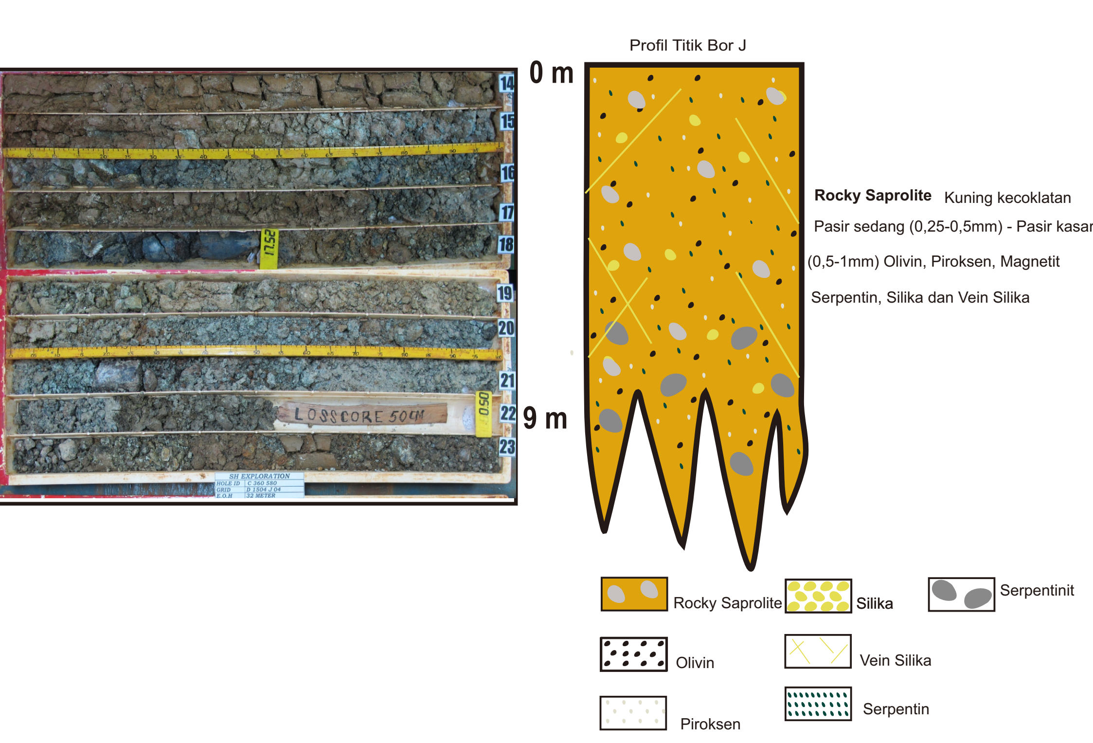
Profil Titik Bor J
