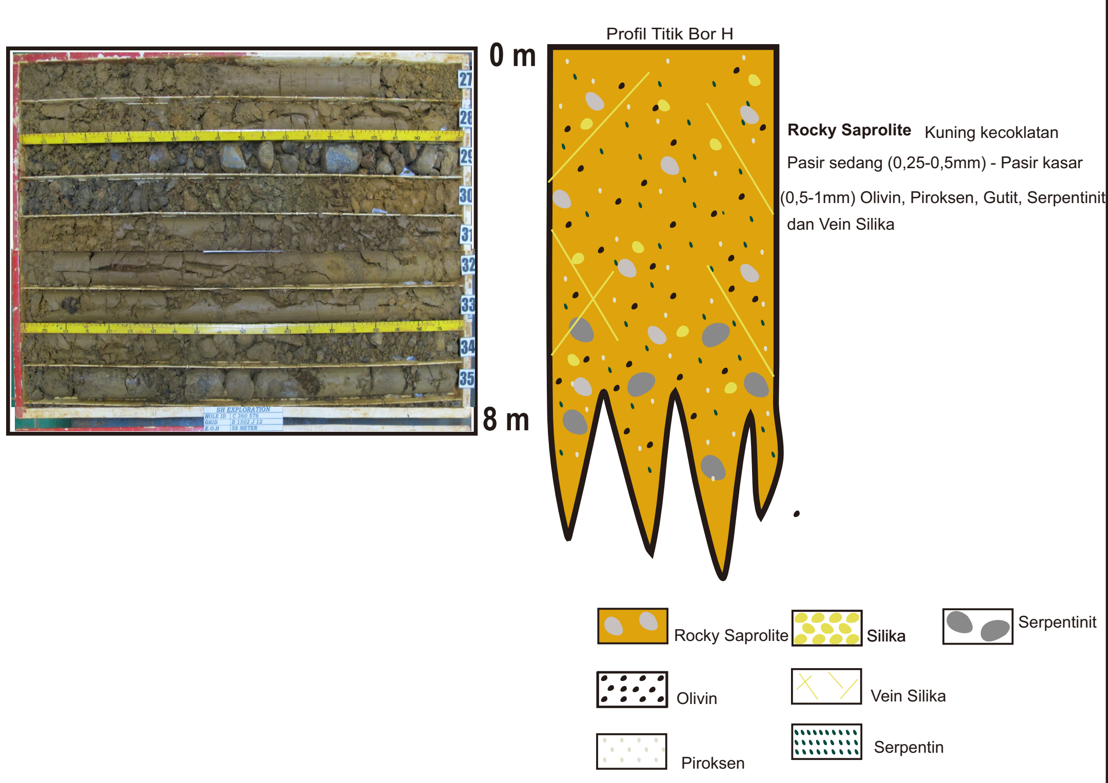
Profil Titik Bor H
