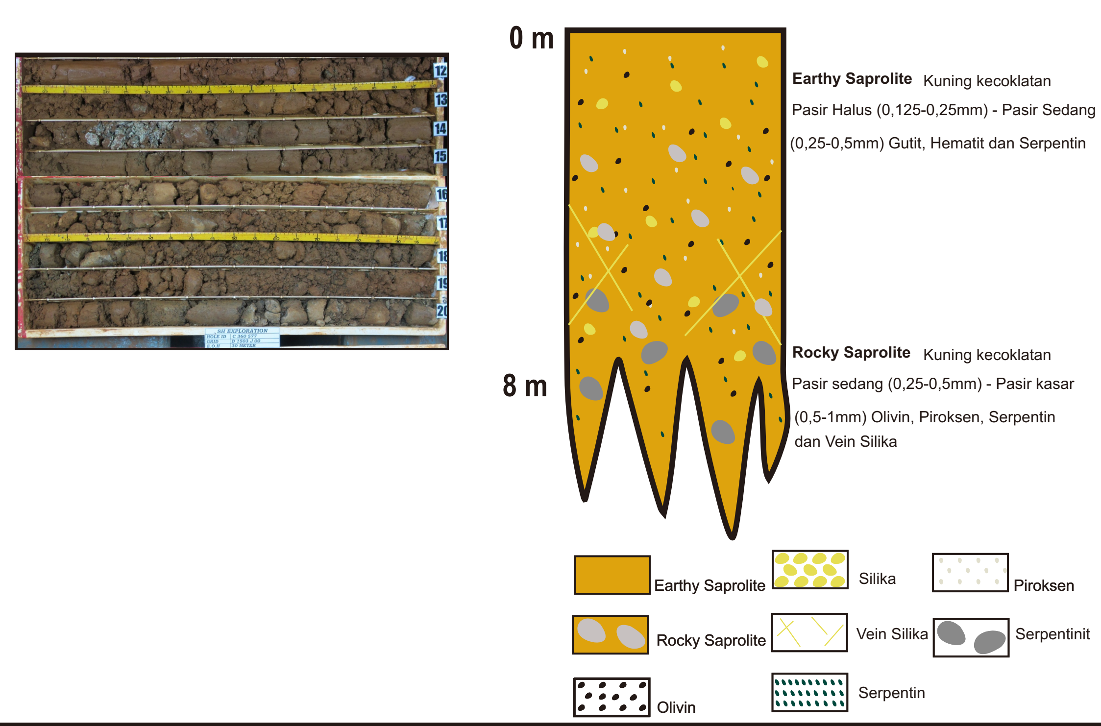
Profil Titik Bor D
