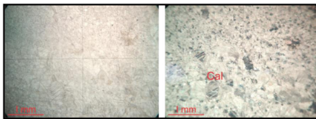
Gambar 7. Sayatan Tipis Batugamping Meta
