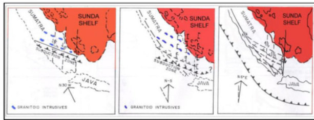
Gambar 1. Tektonik Sumatera (a) Fase Kompresi Jura Awal - Kapur Akhir, (b) Fase Ekstensi Kapur Akhir - Tersier Awal, dan (c) Fase kompresi Miosen Tengah sampai Sekarang (Pulonggono dkk, 1992)
