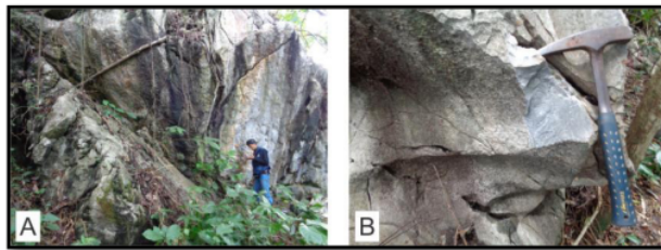
Gambar 2. (A) Singkapan Batugamping Sepingtang Berwarna Hitam, Arah Kamera N 203° E ; (B) Close Up Singkapan, Arah Kamera N 210° E.
