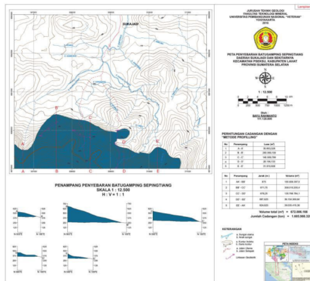
Gambar 8. Peta Sebaran dan Estimasi Cadangan Batugamping Sepingtiang
