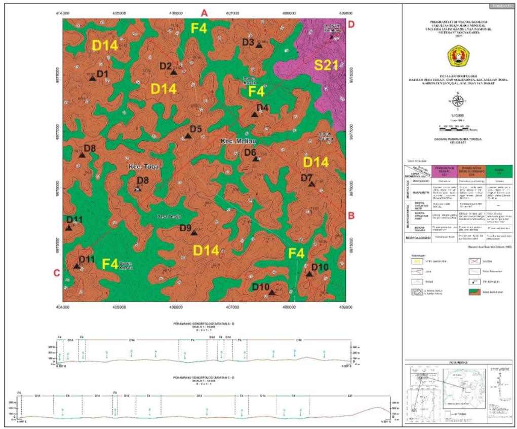
Gambar 1. Peta Geomorfologi
