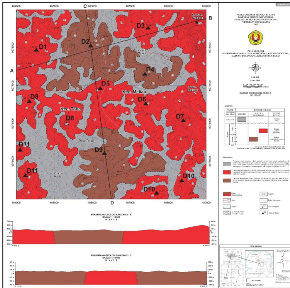
Gambar 3. Peta Geologi
