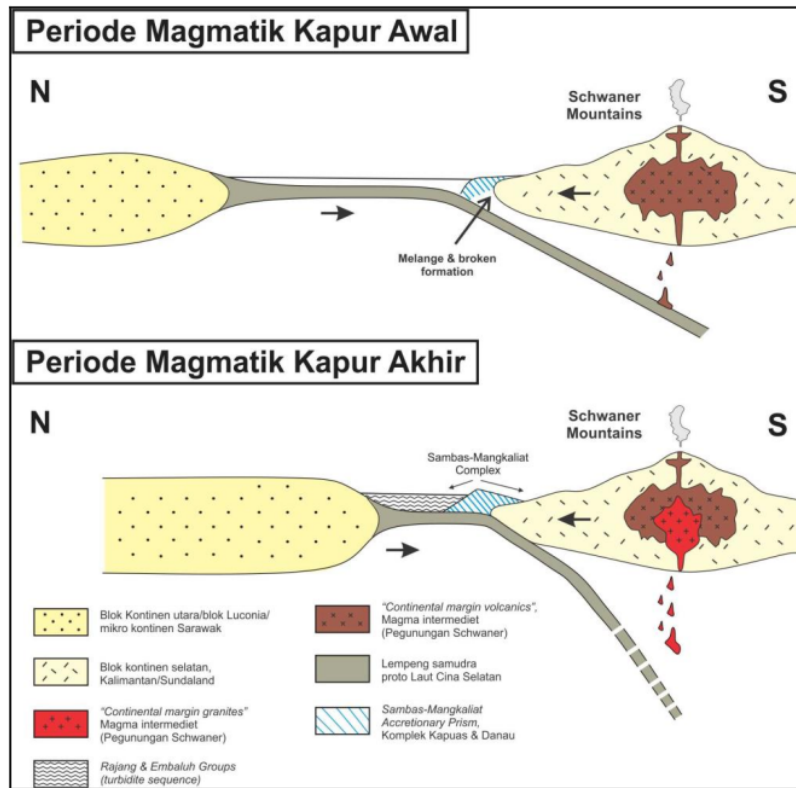
Gambar 5. Sejarah Geologi
