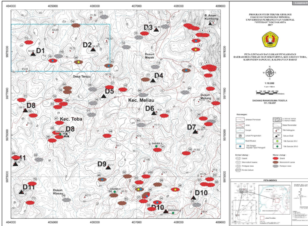
Gambar 2. Peta Lintasan
