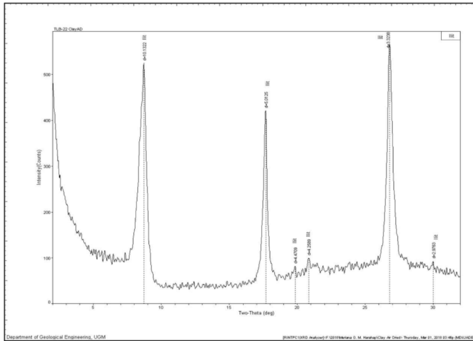
Gambar 10. Grafik analisis XRD clay contoh batuan TLB-22 pada titik LP-54. Terlihat dari grafik terdapat mineral illit.
