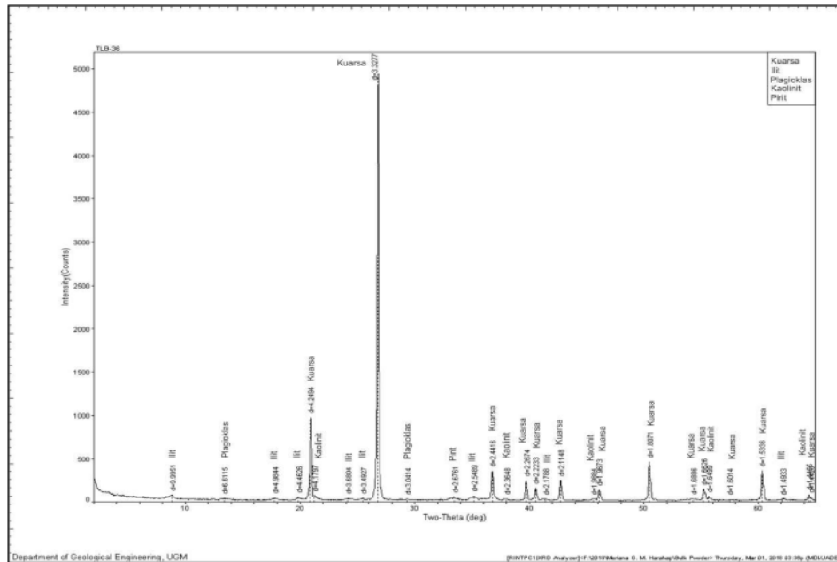
Gambar 13. Grafik analisis XRD bulk conto urat kuarsa TLB-36 pada titik LP-34. Terlihat dari grafik terdapat mineral kuarsa, illit, pagioklas, kaolinit dan pirit. Dominan mineral kuarsa.
