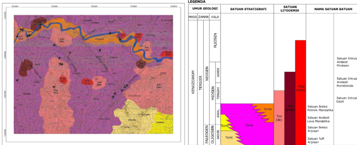
Gambar 14. Peta geologi dan kolom stratigrafi daerah penelitian
