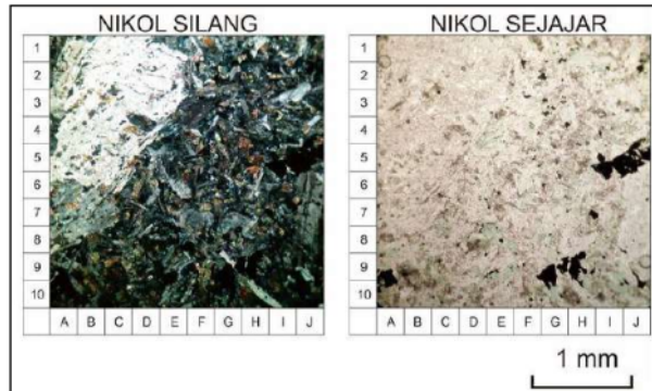
Gambar 20. Foto mikrograf sayatan tipis andesit piroksen pada nikol silang dan nikol sejajar. Contoh sampel TLB-78 pada titik LP-02. Terlihat mineral primer seperti piroksen (H10), palgioklas (J8-J6), dan mineral sekunder seperti Klorit (E9), epidot (G5), mineral opak (A9), yang hadir setempat dalam sayatan petrografi.
