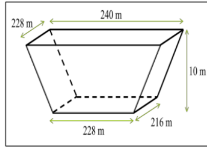
Gambar 11. Dimensi Sump Tahun 2034-2035
