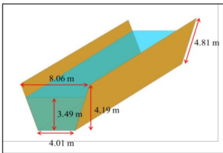
Gambar 7. Dimensi Saluran Terbuka Utara
