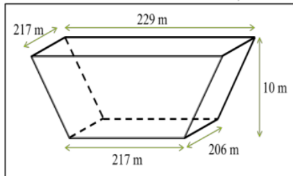
Gambar 10. Dimensi Sump Tahun 2029-2033
