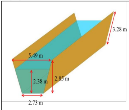
Gambar 6. Dimensi Saluran Terbuka Barat
