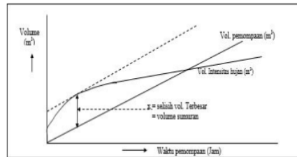
Gambar 1. Grafik Penentuan Volume Sumuran
