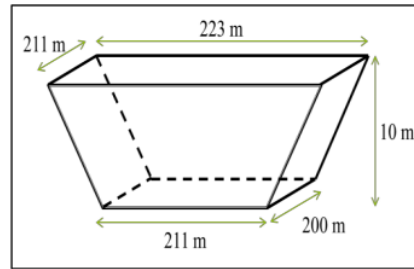
Gambar 8. Dimensi Sump Tahun 2020-2024
