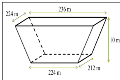
Gambar 12. Dimensi Sump LOM
