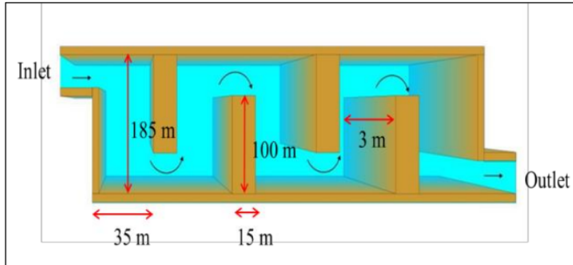
Gambar 15. Dimensi Kolam Pengendapan WMP 14
