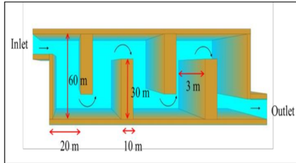
Gambar 13. Dimensi Kolam Pengendapan WMP 11
