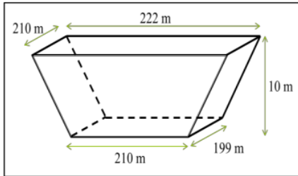
Gambar 9. Dimensi Sump Tahun 2025-2028
