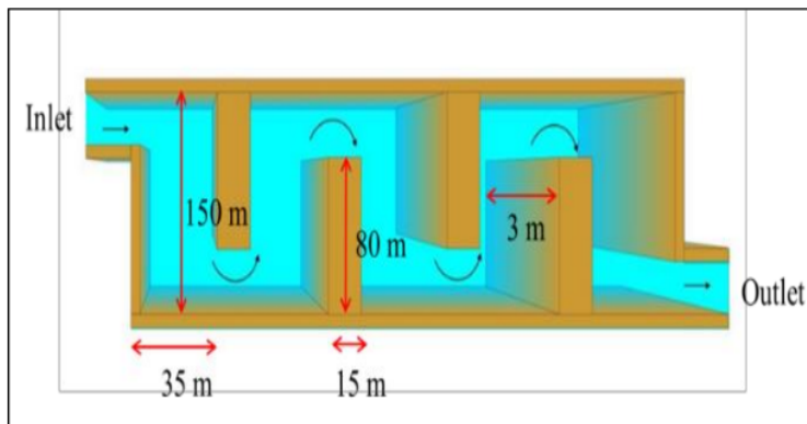
Gambar 16. Dimensi Kolam Pengendapan WMP 15
