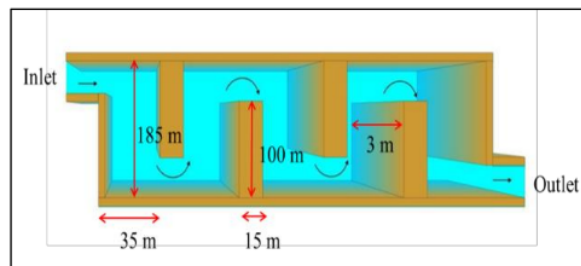
Gambar 14. Dimensi Kolam Pengendapan WMP 13
