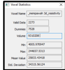
Gambar 4.15. Data Statistik Diorit Masif
