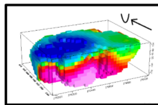
Gambar 4.14. Pemodelan 3D Penampang Resistivitas
