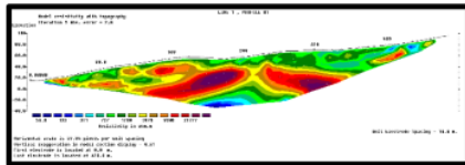
Gambar 4.4. Penampang Resistivitas Lintasan 1
