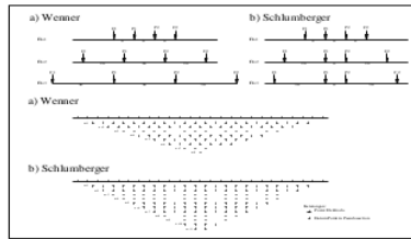
Gambar 3.7. Pengukuran Resistivity dengan konfigurasi elektroda Wenner-Schlumberger
