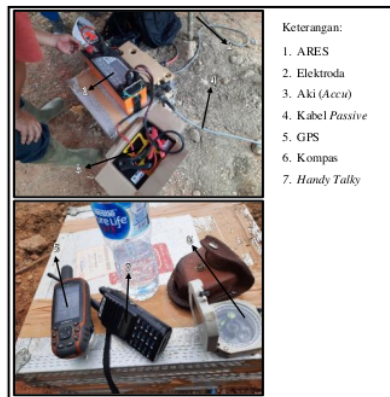
Gambar 4.2. Peralatan dan Perlengkapan
