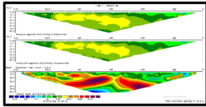
Gambar 4.3. Pemodelan 2D Lintasan 1
