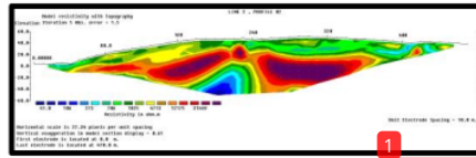
Gambar 4.5. Penampang Resistivitas Lintasan 2
