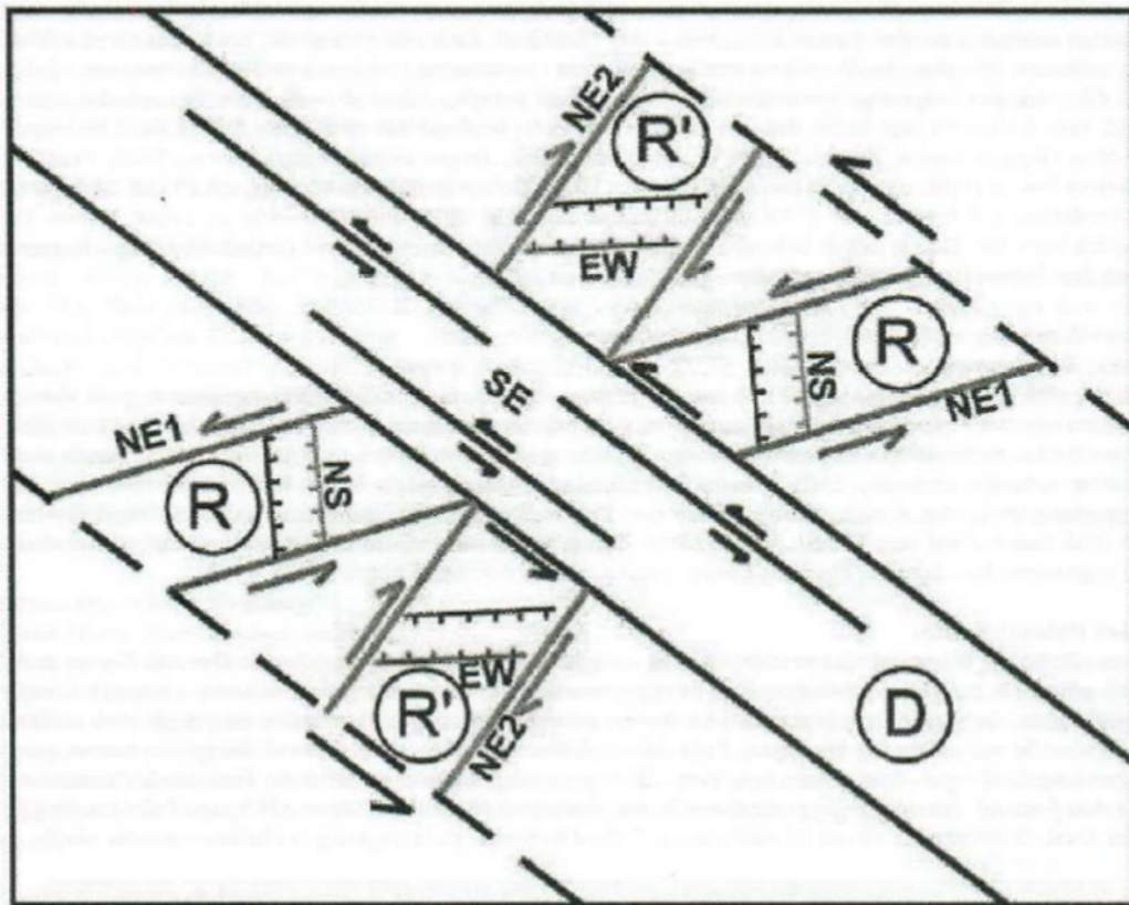
Gambar 2. Model Sesar Pada Daerah Penelitian
