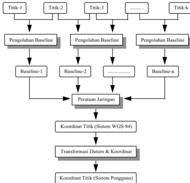
Gambar 8. Diagram alir perhitungan koordinat titik-titik jaringan GPS
