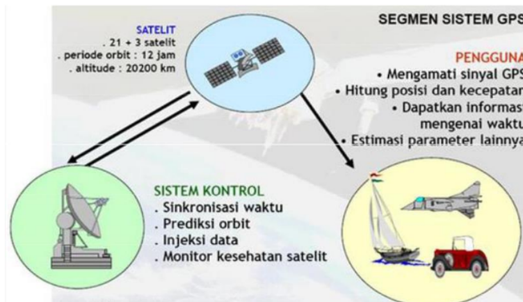
Gambar 2. Sistem penentuan posisi GPS (Abidin, 1995)
