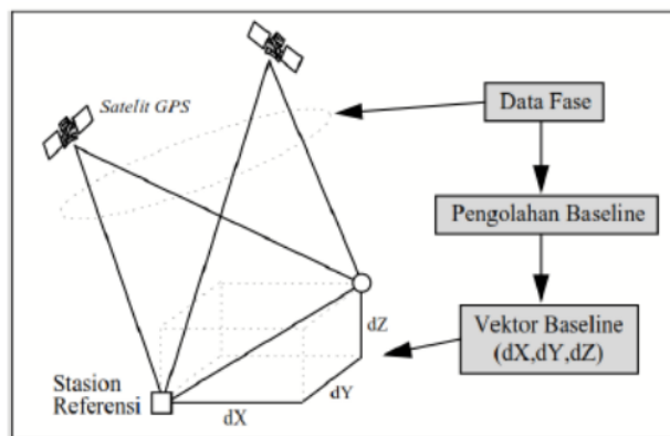
Gambar 15. Pengolahan data baseline GNSS (SNI JKH, 2002)
