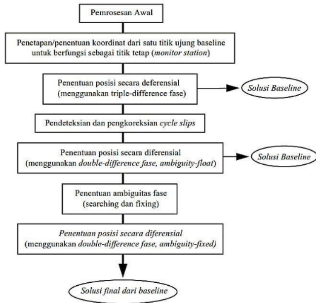
Gambar 16. Tahapan perhitungan suatu baseline GNSS (SNI JKH, 2002)
