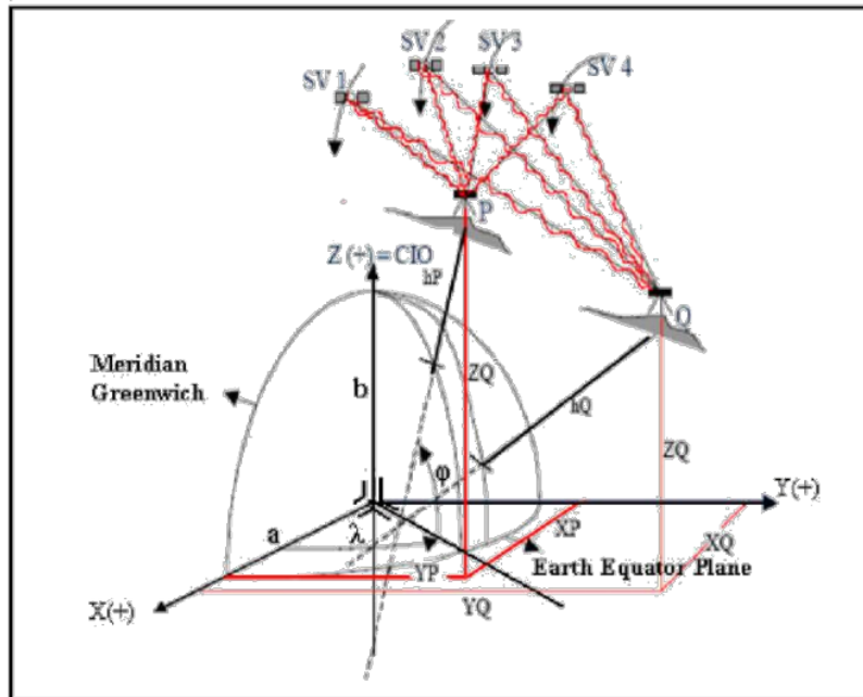
Gambar 6. Penentuan posisi relatif pengamatan GPS (Widjajanti, 2010)
