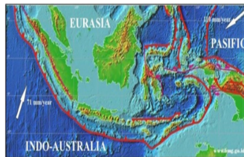
Gambar 2. Pertemuan tiga lempeng lithosfer kepulauan Indonesia
