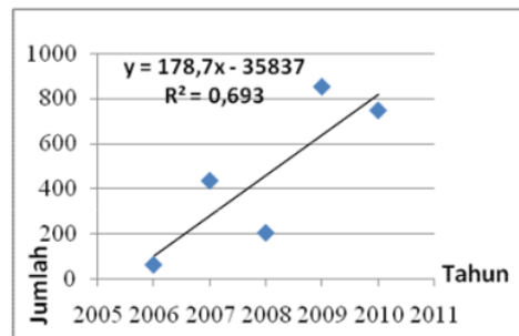
Gambar 8. Regresi linier sederhana intensitas gempa bumi di Indonesia periode tahun 2006 – 2010
