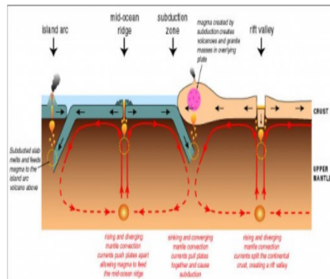
Gambar 6. Pergerakan konveksi dari magma
