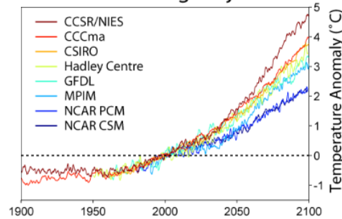
Gambar 4. Perhitungan pemanasan global pada tahun 2001 dari beberapa model iklim berdasarkan scenario SRES(Special Report on Emissions Scenarios) A2, yang mengasumsikan tidak ada tindakan yang dilakukan untuk mengurangi emisi.
