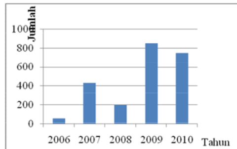
Gambar 7. Grafik gempa bumi dengan magnetometer diatas 5,0 skala Richter periode tahun 2006 – 2010 di Indonesia
