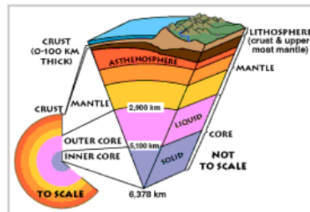
Gambar 5. Struktur Bumi
