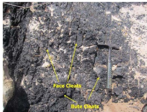
Gambar 4. Kenampakan Face Cleats dan Bute Cleats Seam M-10 Formasi Warukin
