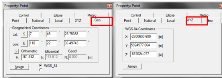
Gambar 28. Pendefinisian koordinat titik fixed
