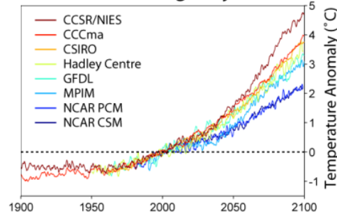
1 Gambar 4. Perhitungan pemanasan global pada tahun 2001 dari beberapa model iklim berdasarkan scenario SRES(Special Report on Emissions Scenarios) A2, yang mengasumsikan tidak ada tindakan yang dilakukan untuk mengurangi emisi.
