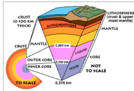
Gambar 5. Struktur Bumi
