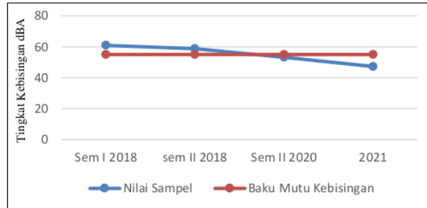
Gambar 3. Grafik Hasil Pengukuran Kebisingan dengan Baku Mutu Sumber: Dokumentasi Pelaksanaan RKL/RPL UP. Pamo dan Olah Data (2021)
