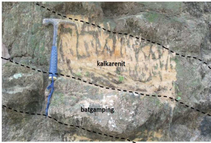
Gambar 3.9. Kalkarenit sisipan batugamping, berlapis dan massif, kedudukan relatif horizontal, pada Satuan Kalkarenit Ledok. (MAF)
