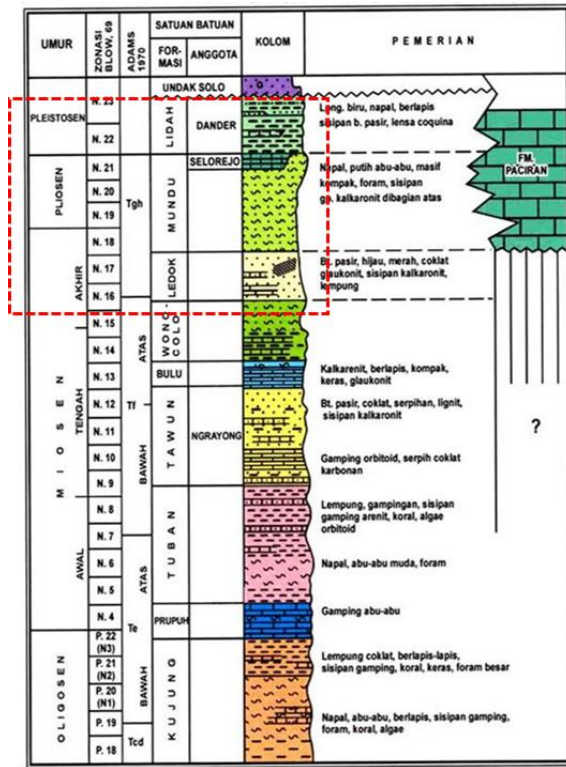
Gambar 3.3. Kolom Stratigrafi Zona Rembang (Pringgoprawiro, 1983)
