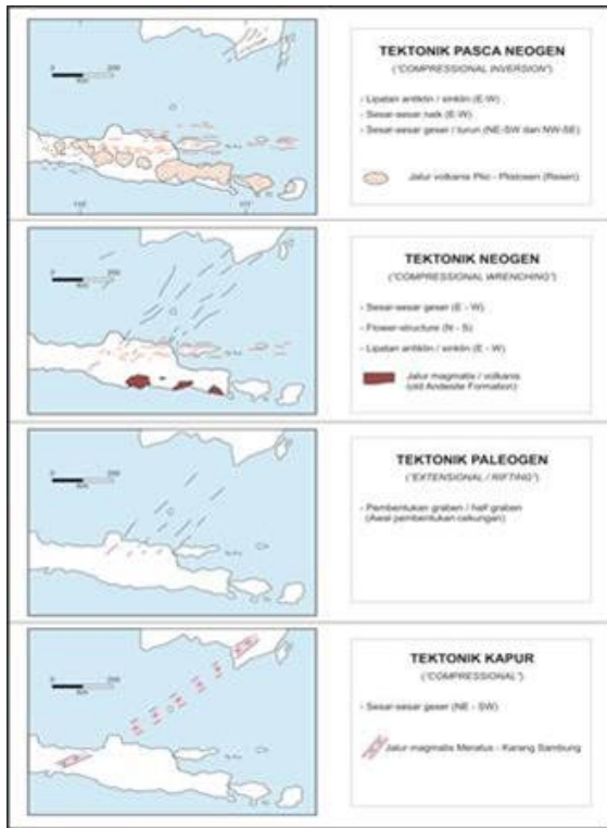
Gambar 3.2 Evolusi Tektonik Cekungan Jawa Timur Utara (Lemigas, 2003)
