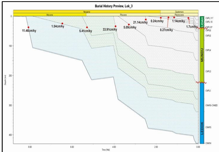
Gambar 5.14 Kurva model burial history Lokasi Kedewan
