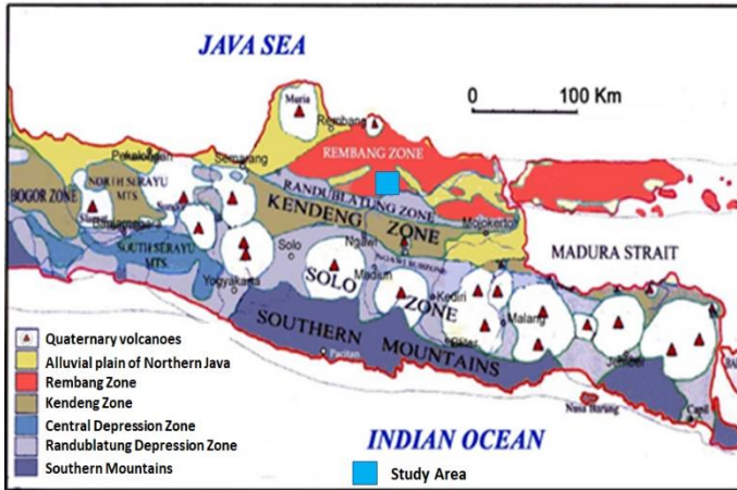
Gambar 1.2. Fisiografi Cekungan Jawa Tiur Utara (van Bemmelen, 1949).
