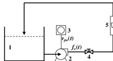
Gambar 1. Rangkaian alat percobaan.
