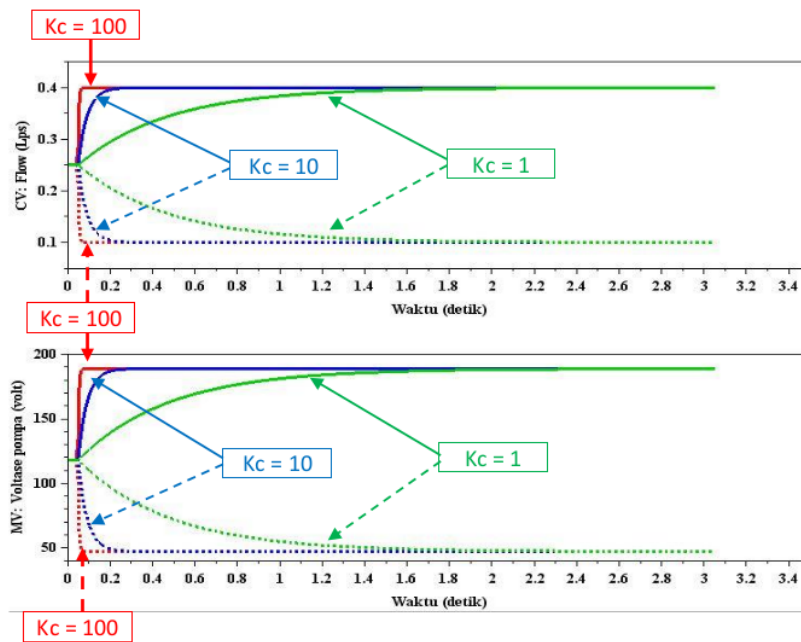
Gambar 8. Respon dinamis loop tertutup terhadap perubahan set point \Delta f = \pm 0.15 L/detik dengan \tau_i = 0,01 detik dan variasi K_c = 1, 10, 100 [L/(volt.detik)].
