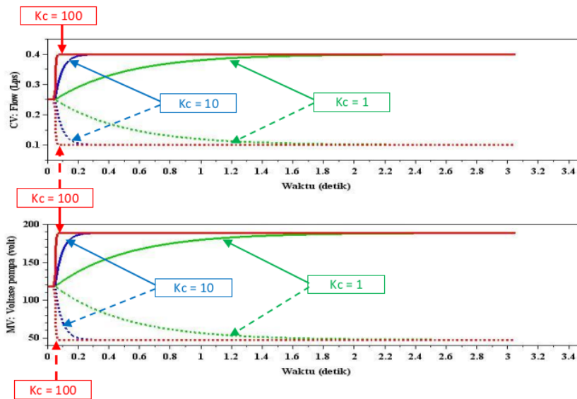
Gambar 7. Respon dinamis loop tertutup terhadap perubahan set point \Delta f = \pm 0.15 L/detik dengan \tau_i = 0,1 detik dan variasi K_c = 1, 10, 100 [L/(volt.detik)].
