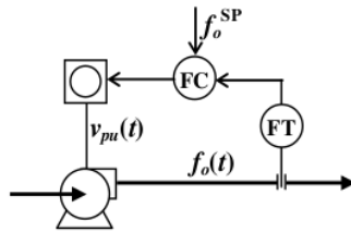
Keterangan: FT: Flow Transmitter; FC: Flow Controller Gambar 2. Usulan konfigurasi pengendalian laju alir cairan.
