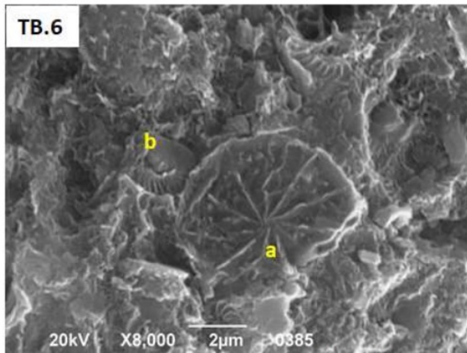
a) Hayaster perplexus
