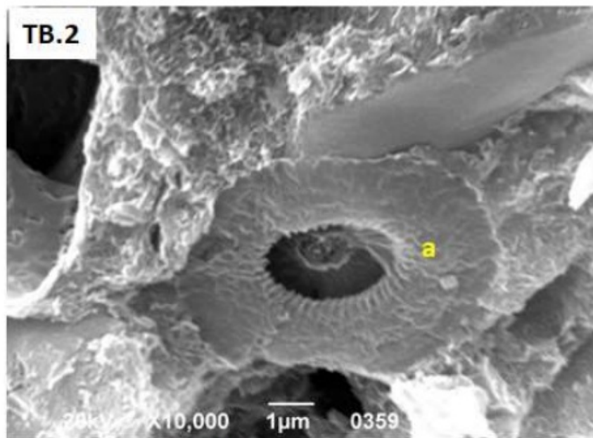
a) Calcidiscus macintyreii
