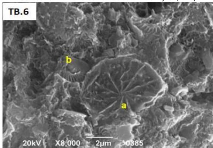
a) Hayaster perplexus
