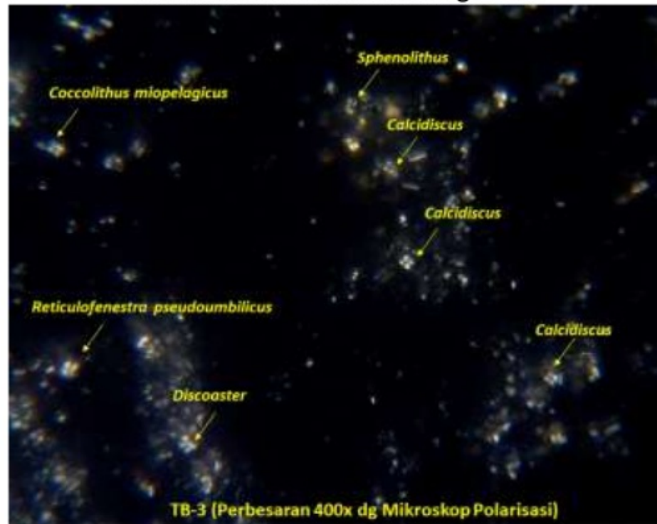
Gambar 5.4. Nannofossil berdasarkan pengamatan menggunakan mikroskop polarisasi dengan perbesaran (400x) pada sampel Tb.3
