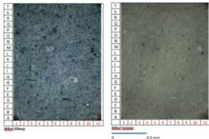
Gambar 3.7. Sayatan petrografi sampel 7-TB.6
