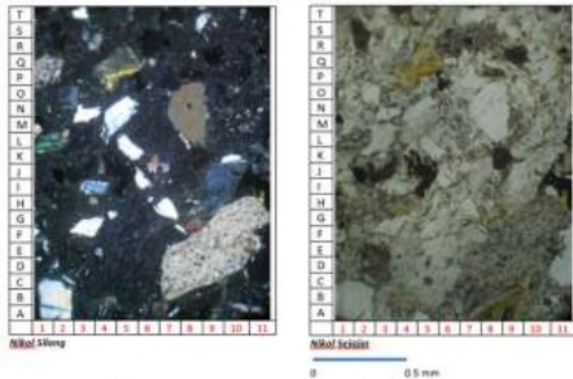
Gambar 3.6. Sayatan petrografi sampel 6-TB.4
