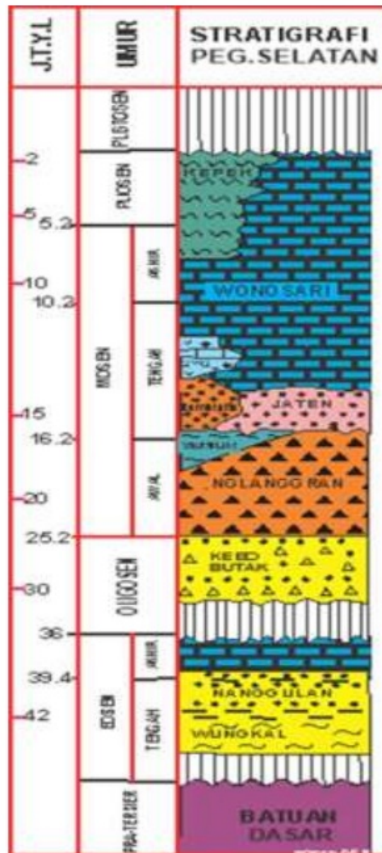
Gambar 2.2. Stratigrafi Pegunungan Selatan (Surono, 1992)
