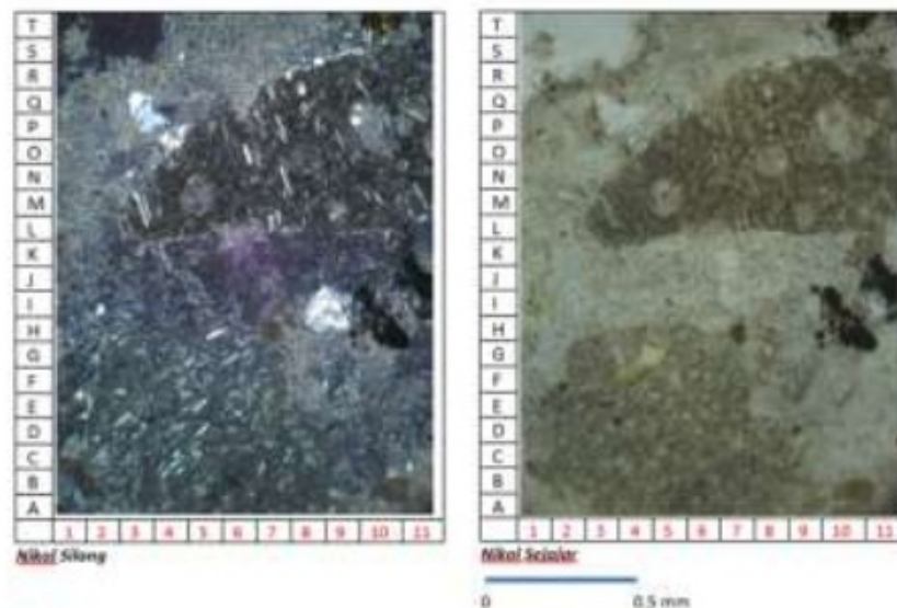
Gambar 3.4. Sayatan petrografi sampel 3-TB.3
