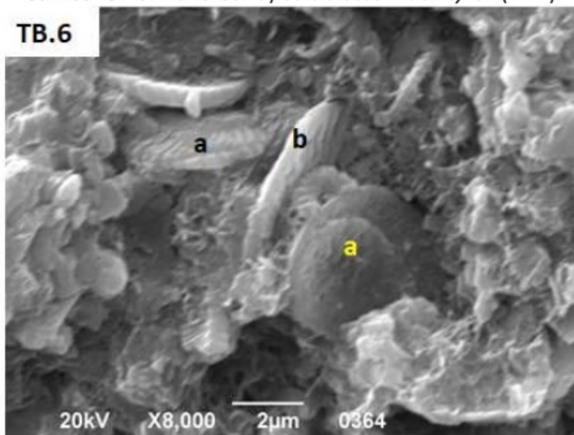
a) Coccolithus miopelagicus b) Calcidiscus macintyreii
