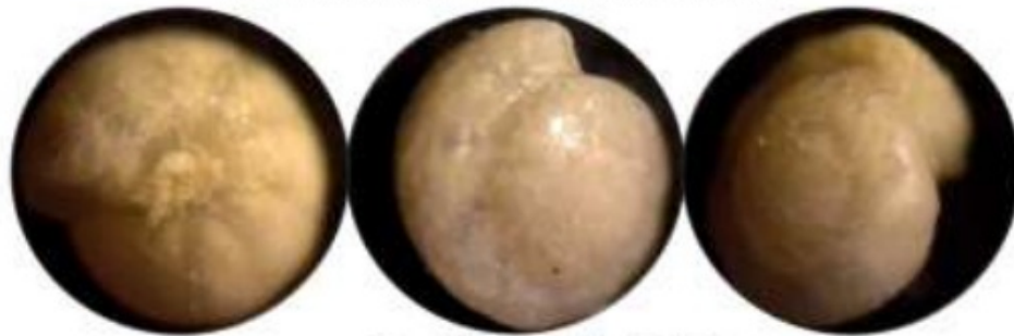
Gyroidina neosoldanii 1450 ftm
