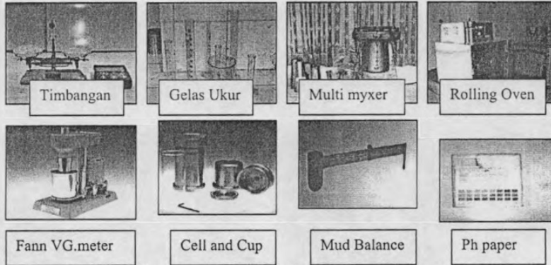
Gambar 4. Peralatan Ukur dan Pengujian Laboratorium Lumpur Bor.
