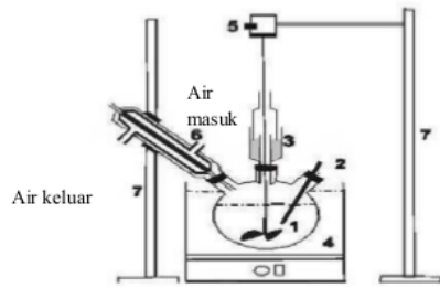
Gambar 2: Rangkaian alat hidrolisis
