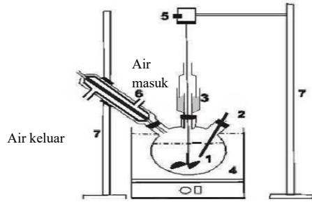
Gambar 2: Rangkaian alat hidrolisis
