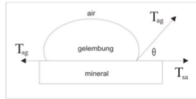
Gambar 3. Sudut kontak antara mineral-udara dan air.
