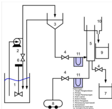
Gambar 6. Rangkaian Alat yang Digunakan
