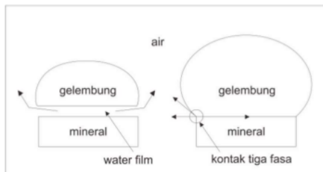
Gambar 2. Skematika Pelekatan Mineral – Gelembung
