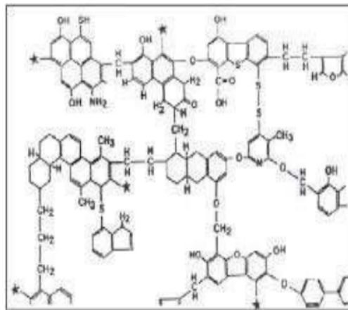
Gambar 1. Struktur batubara model Wisser (Krevelen, 1993)
