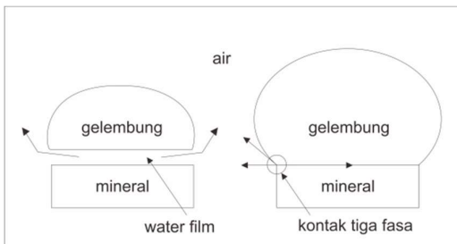
Gambar 2. Skematika Pelekatan Mineral – Gelembung
