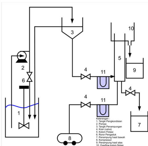
Gambar 6. Rangkaian Alat yang Digunakan
