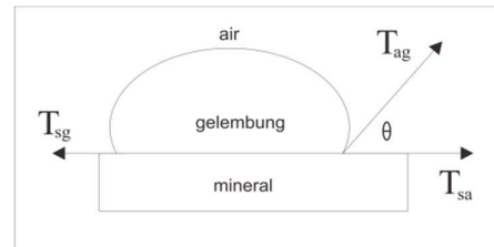
Gambar 3. Sudut kontak antara mineral-udara dan air.
