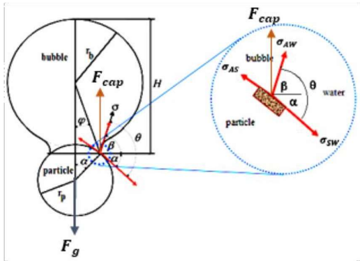
Gambar 4. Geometri axisymmetric partikel melekat bawah gelembung (Nguyen, 2003)
