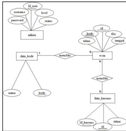
Gambar 4. ERD
