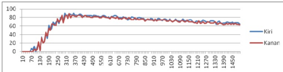
Gambar 18 grafik pengujian dengan set point 50 konstanta proportional 0.4
