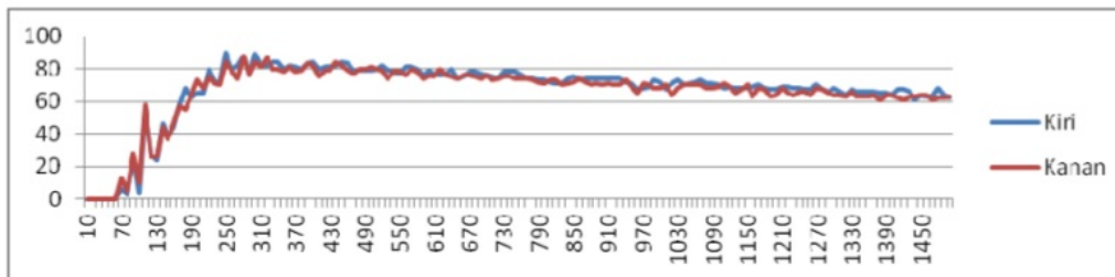
Gambar 20 grafik pengujian dengan set point 50 konstanta proportional 0.6
