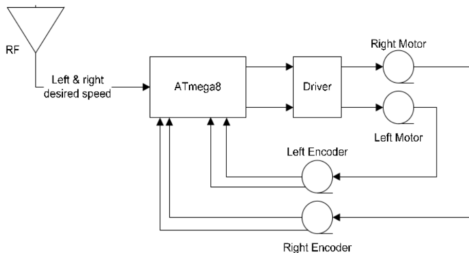
Gambar 2 Blok diagram sistem robot mirosot
