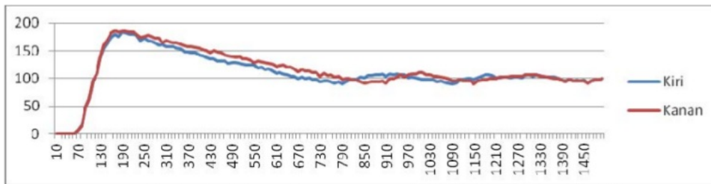
Gambar 7 grafik pengujian dengan set point 100 konstanta proportional 0.3
