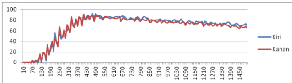
Gambar 16 grafik pengujian dengan set point 50 konstanta proportional 0.2
