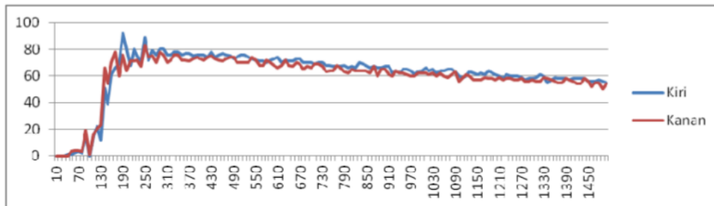
Gambar 23 grafik pengujian dengan set point 50 konstanta proportional 0.9
