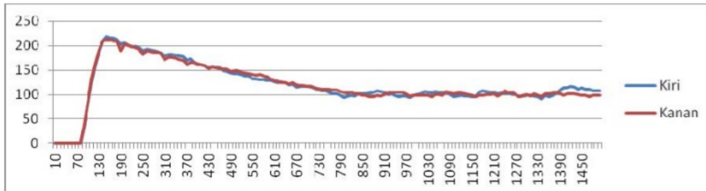
Gambar 11 grafik pengujian dengan set point 100 konstanta proportional 0.7
