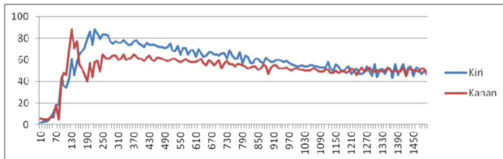
Gambar 24 grafik pengujian dengan set point 50 konstanta proportional 1.0
