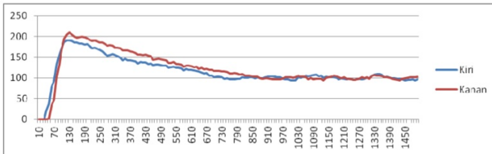
Gambar 10 grafik pengujian dengan set point 100 konstanta proportional 0.6
