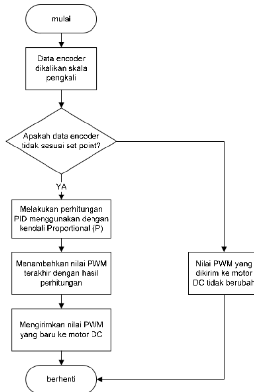
Gambar 4 Flowchart kendali kecepatan atau fungsi mcontrol()
