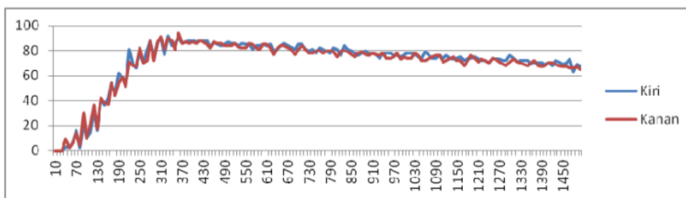
Gambar 17 grafik pengujian dengan set point 50 konstanta proportional 0.3
