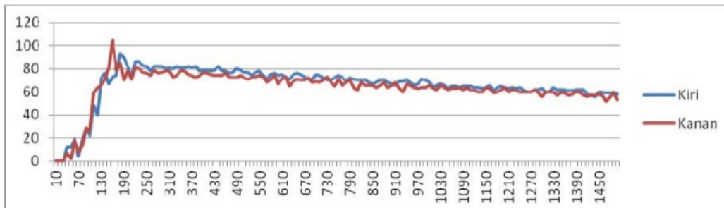
Gambar 21 grafik pengujian dengan set point 50 konstanta proportional 0.7
