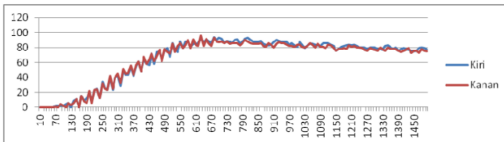
Gambar 15 grafik pengujian dengan set point 50 konstanta proportional 0.1
