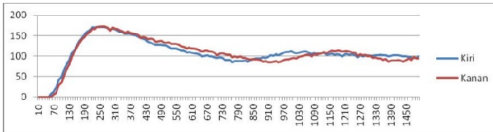
Gambar 5 grafik pengujian dengan set point 100 konstanta proportional 0.1
