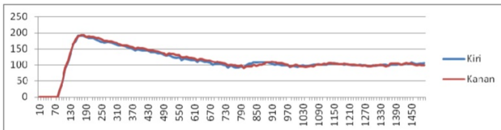
Gambar 8 grafik pengujian dengan set point 100 konstanta proportional 0.4
