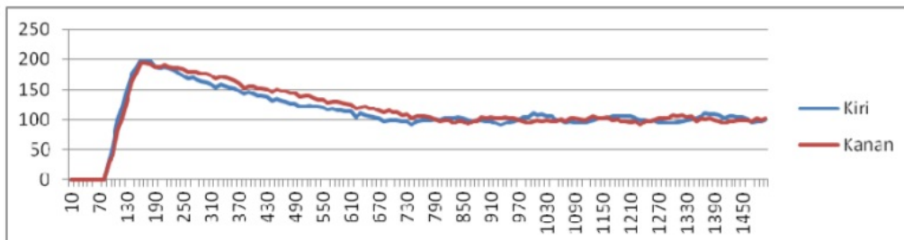
Gambar 9 grafik pengujian dengan set point 100 konstanta proportional 0.5
