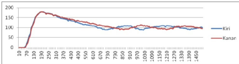
Gambar 6 grafik pengujian dengan set point 100 konstanta proportional 0.2
