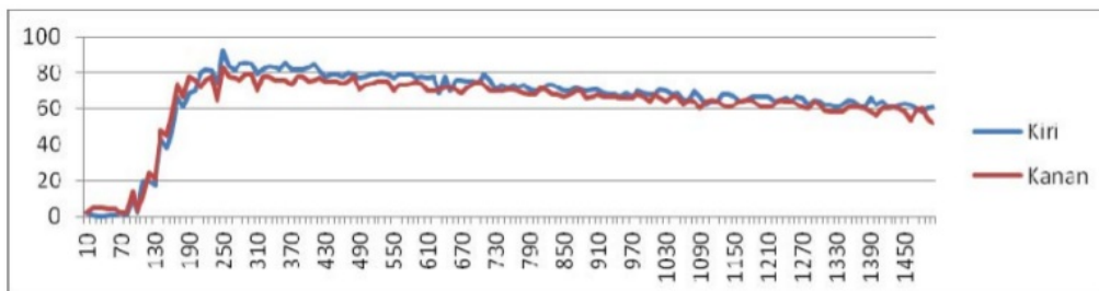
Gambar 22 grafik pengujian dengan set point 50 konstanta proportional 0.8
