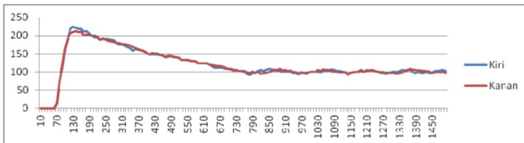
Gambar 13 grafik pengujian dengan set point 100 konstanta proportional 0.9
