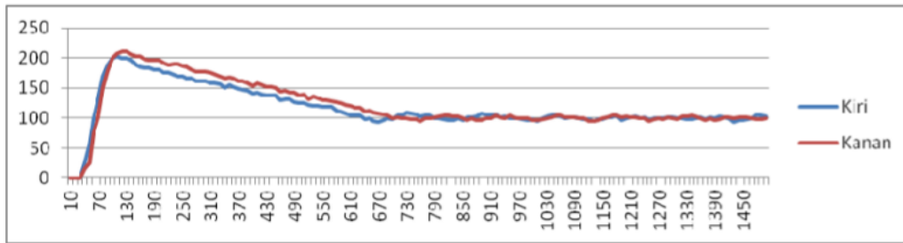
Gambar 143 grafik pengujian dengan set point 100 konstanta proportional 1.0
