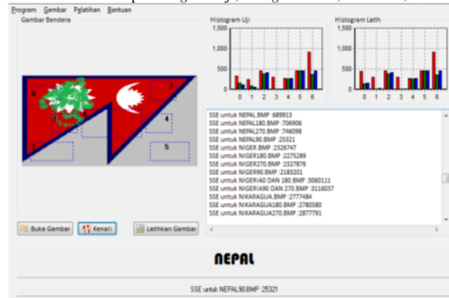
Gambar 4.6 Form Pengujian
