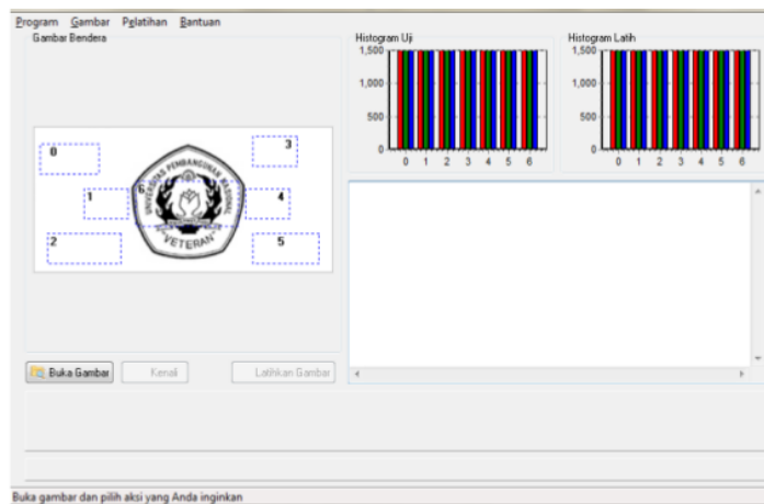
Gambar 6 Form Utama
