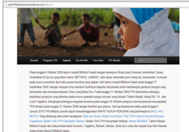
Gambar 2. Pengantar Web
