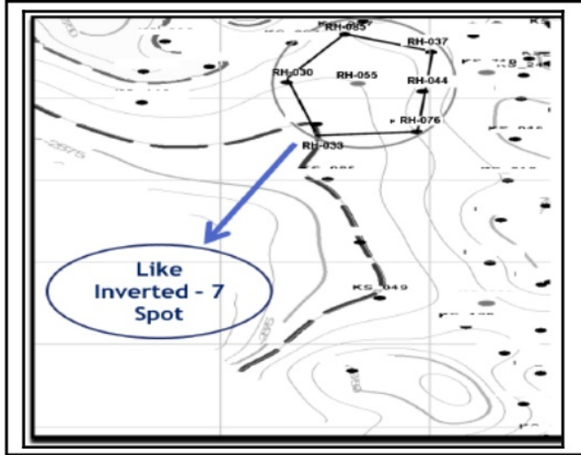
Gambar C. Pola Sumur Injeksi-Produksi Lapangan "A"
