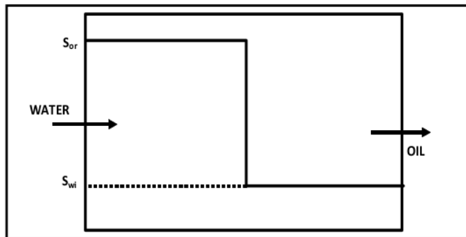
Gambar B. Konsep Pendesakan Piston Like Displacement
