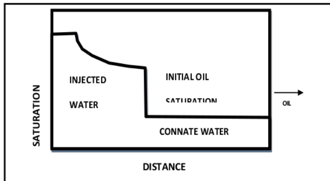
Gambar A. Konsep Pendesakan Desaturasi
