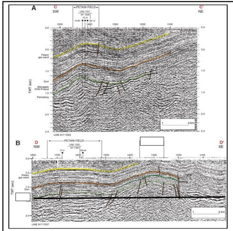
Gambar G. Struktur Geologi Lapangan
