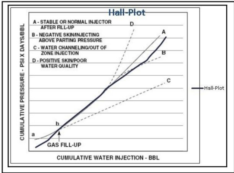
Gambar F. Kurva Hall-Plot Sumur Injeksi
