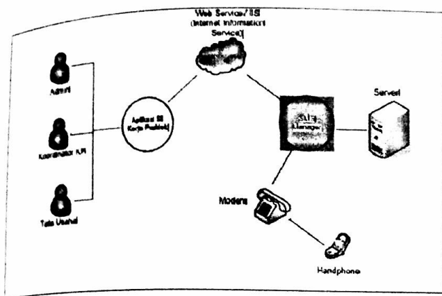
Gambar 1 Arsitektur Sistem
