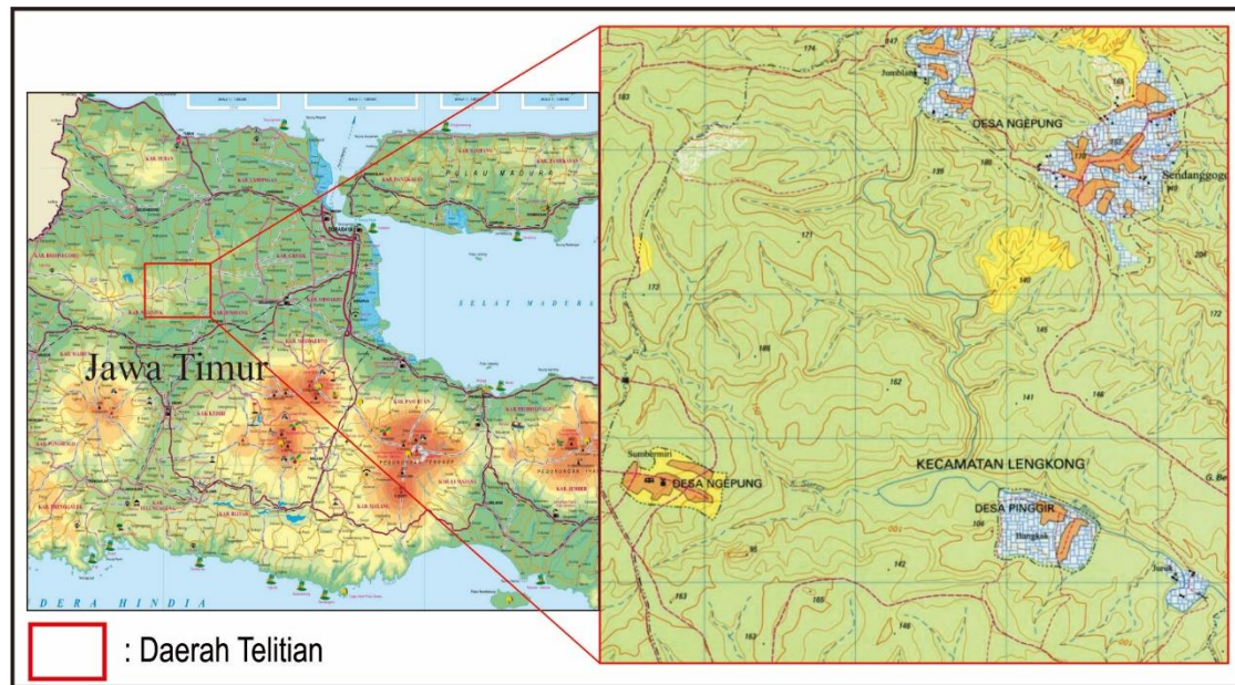
Gambar 1: Peta lokasi penelitian daerah Pinggir dan sekitarnya, Kecamatan Lengkung, Kabupaten Nganjuk, Jawa Timur
